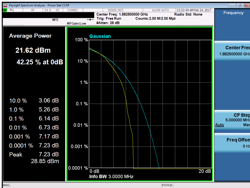
Plot 7-165. PAR Plot (Band 25/2 – 3.0MHz 16-QAM – RB Size 15)
