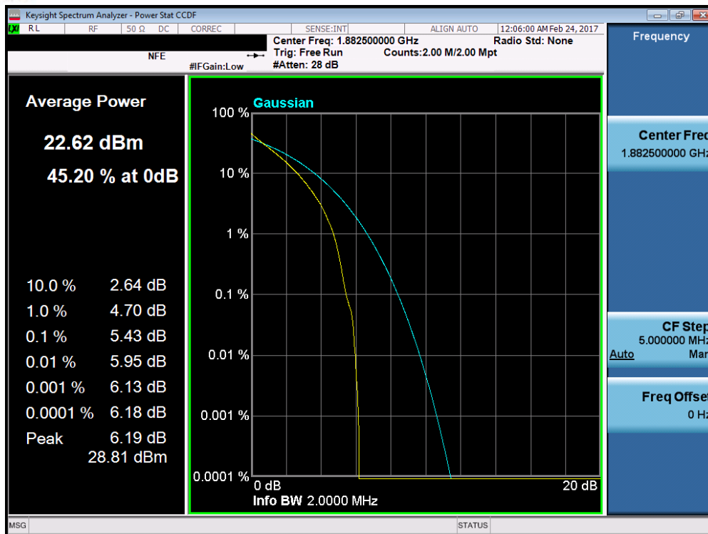
Plot 7-162. PAR Plot (Band 25/2 – 1.4MHz QPSK – RB Size 6)
