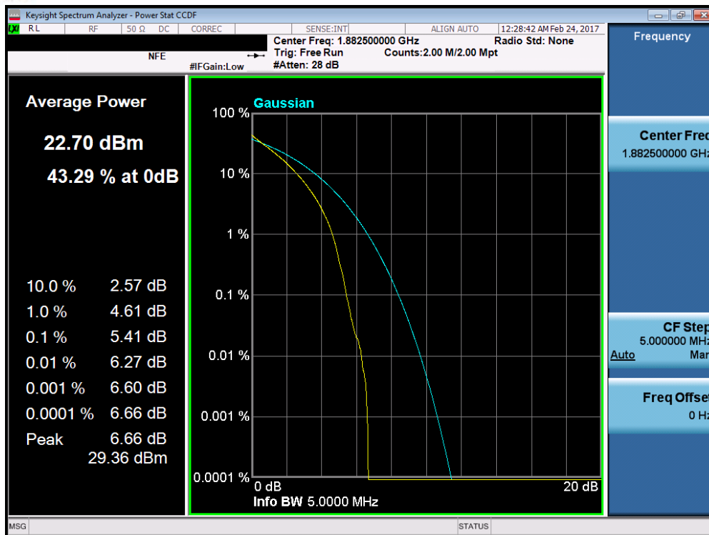
Plot 7-166. PAR Plot (Band 25/2 – 5.0MHz QPSK – RB Size 25)
