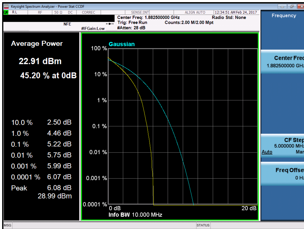
Plot 7-168. PAR Plot (Band 25/2 – 10.0MHz QPSK – RB Size 50)
