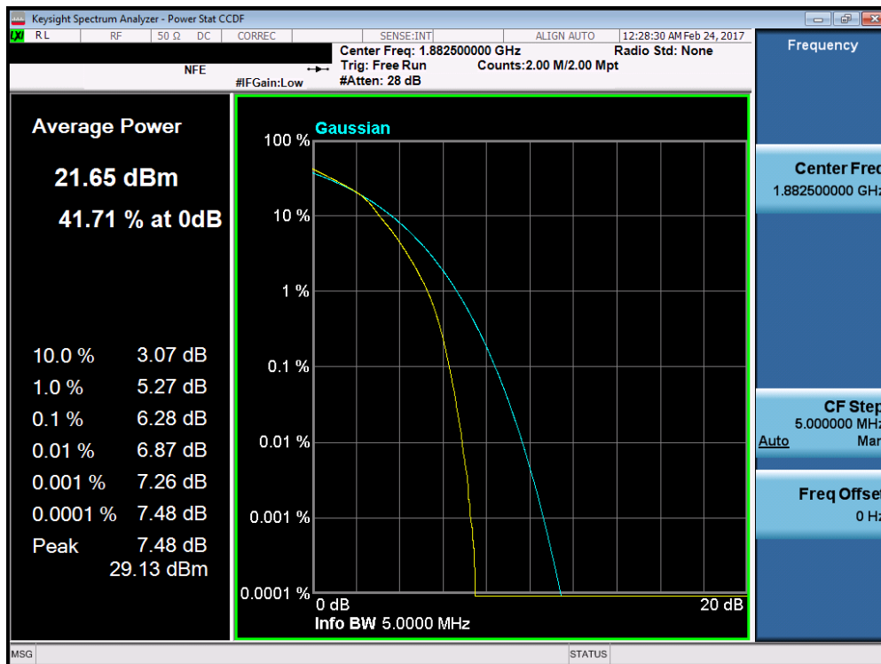
Plot 7-167. PAR Plot (Band 25/2 – 5.0MHz 16-QAM – RB Size 25)
