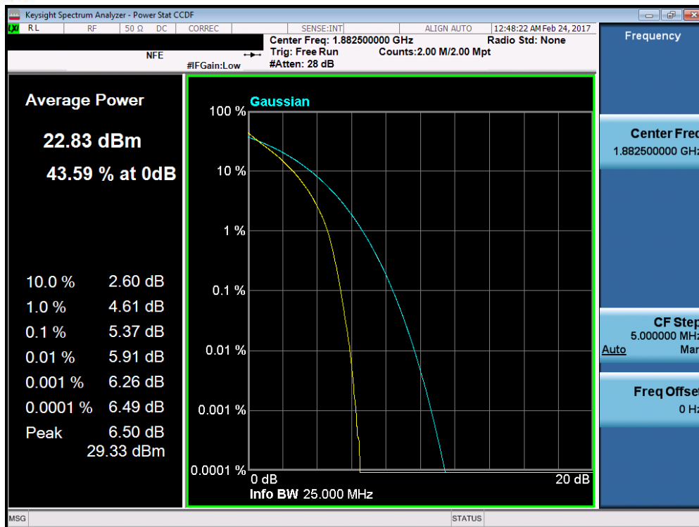
Plot 7-172. PAR Plot (Band 25/2 – 20.0MHz QPSK – RB Size 100)
