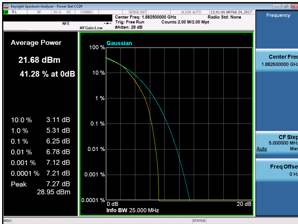
Plot 7-171. PAR Plot (Band 25/2 – 15.0MHz 16-QAM – RB Size 75)
