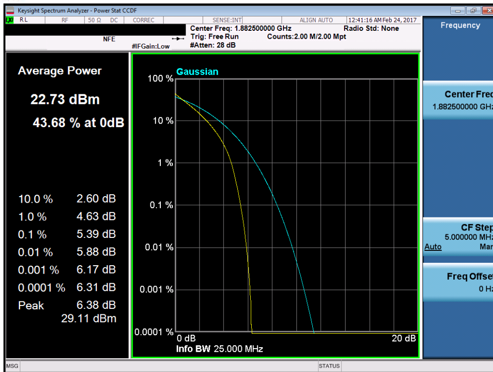
Plot 7-170. PAR Plot (Band 25/2 – 15.0MHz QPSK – RB Size 75)
