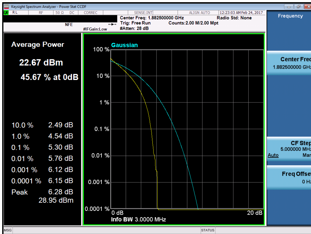
Plot 7-164. PAR Plot (Band 25/2 – 3.0MHz QPSK – RB Size 15)
