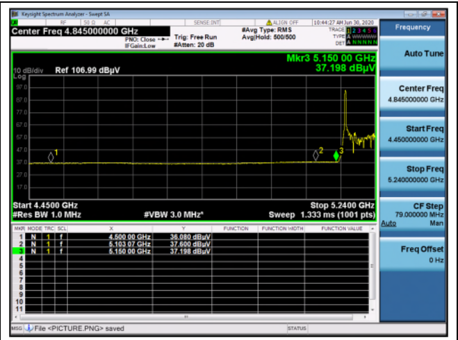
Middle channel_0 RU (Average)
