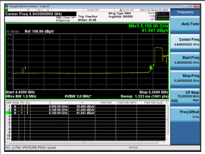
Middle channel_65 RU (Average)
