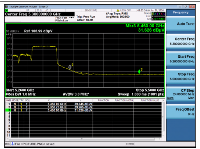
Middle channel_66 RU (Average)
