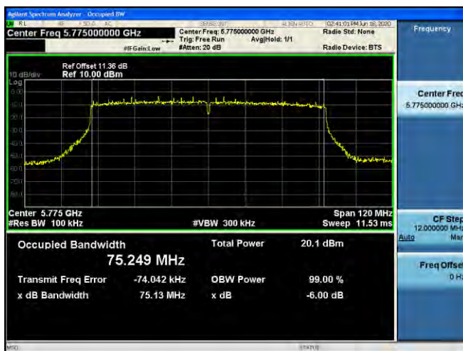
802.11ac(VHT80) (CH.155)
