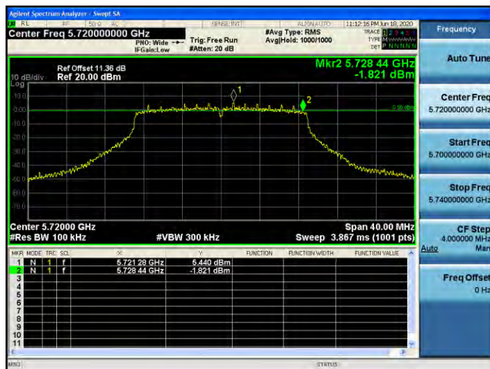
802.11n_HT20 CH.144
