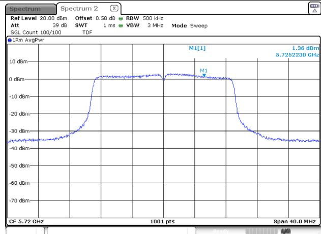
UNII-3 / 802.11n HT40
