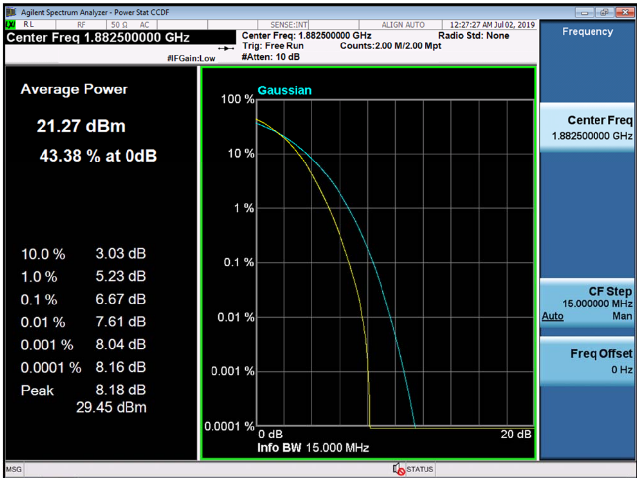
BAND 25/2. PAR Plot (15M BW Ch.26365 64QAM RB 75_0)
