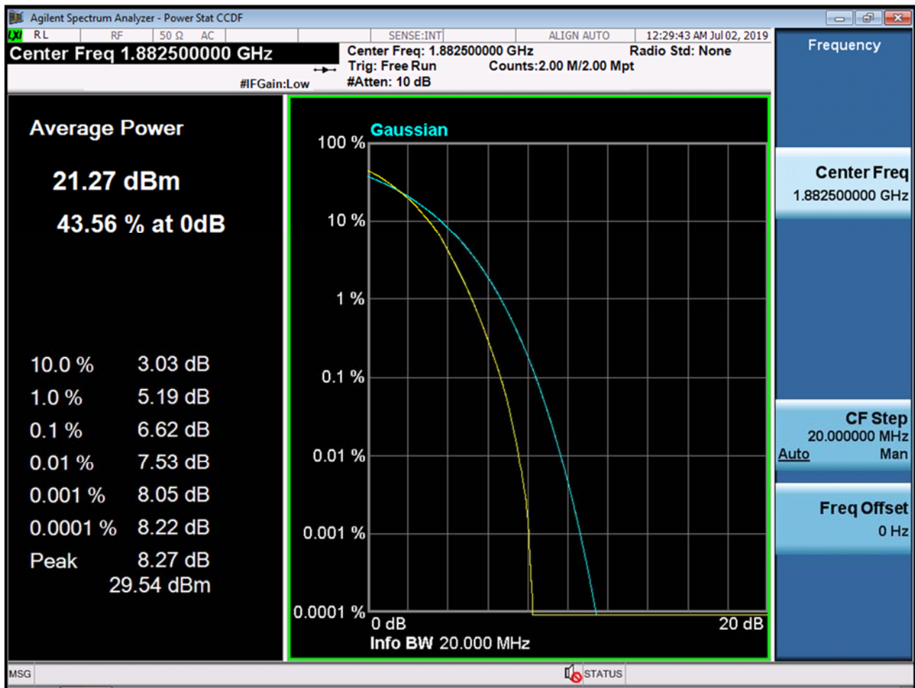
BAND 25/2. PAR Plot (20M BW Ch.26365 64QAM RB 100_0)
