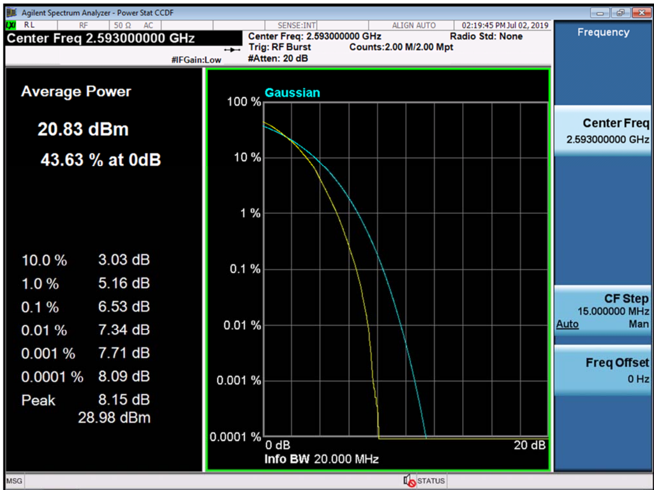
BAND 41. PAR Plot (20M BW_Ch.40620_64QAM_RB100_0)
