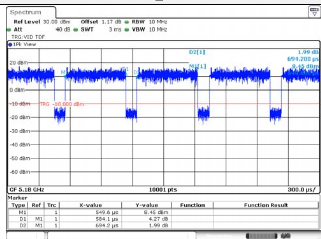
802.11ax_HE20 / SU
