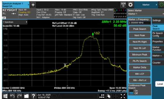
8DPSK Band Edge(Ch. 0)
