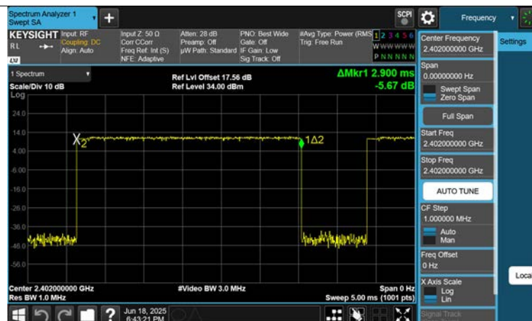
\pi/4 DQPSK : Dwell Time(Ch. 0)
