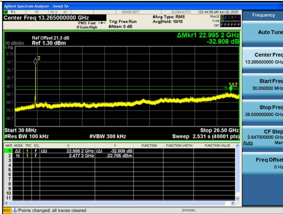
[ANT. 2] 802.11g_Ch.13
