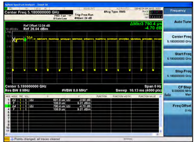
802.11ac(VHT20)
