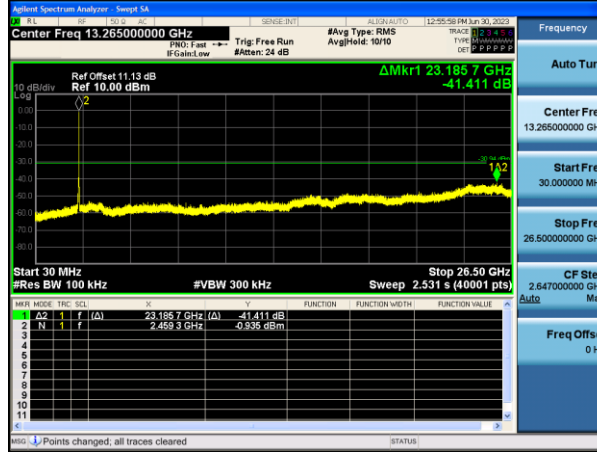
[MIMO ANT. 1] 802.11g Ch.11 18 Mbps
