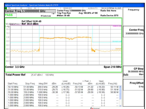
5G NR n77 100MHz BPSK Mid Channel RB270-0
