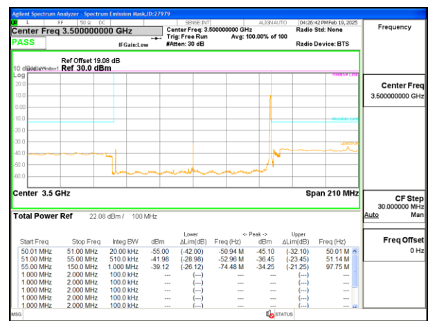
5G NR n77 100MHz BPSK Mid Channel RB1-272
