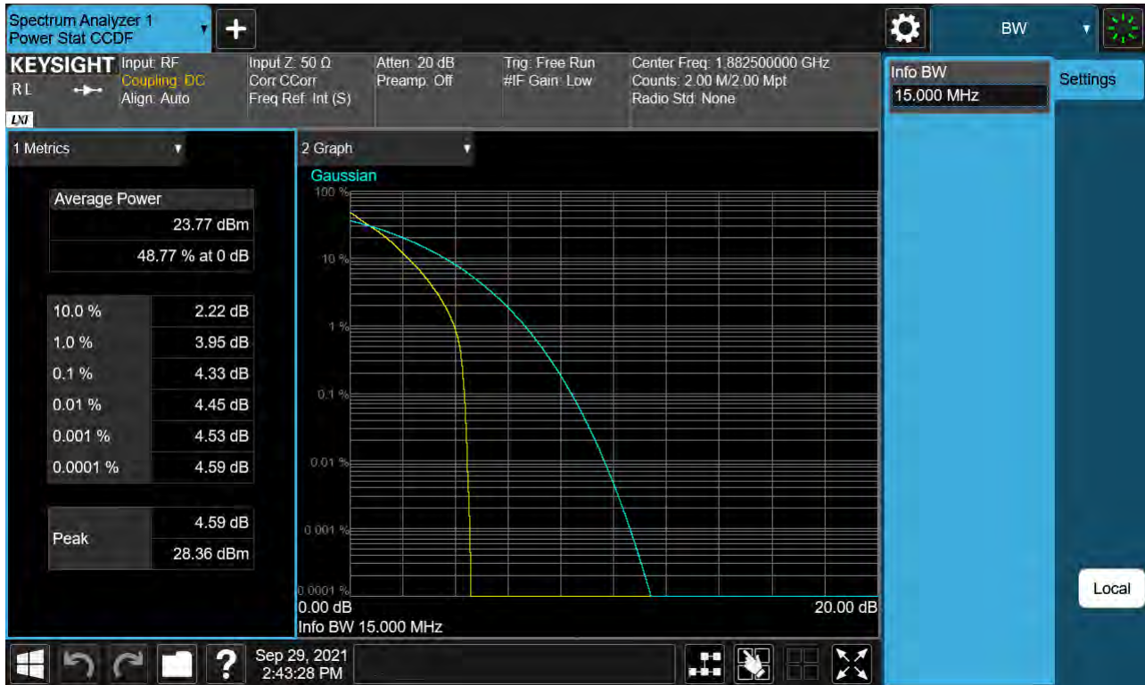
Sub6 n25(2). PAR Plot (15 M BW Ch.376500 QPSK _ Full RB _0)
