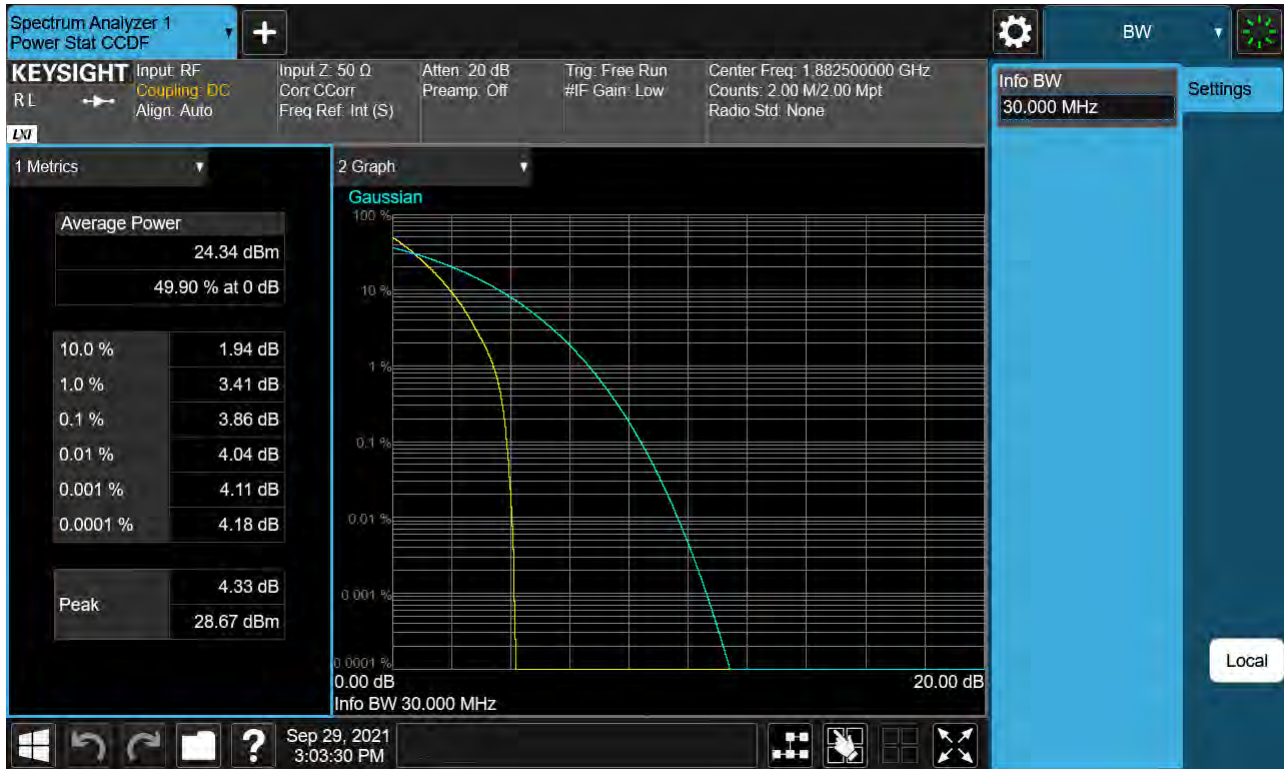
Sub6 n25. PAR Plot (30 M BW Ch.376500 BPSK_ Full RB _0 )
