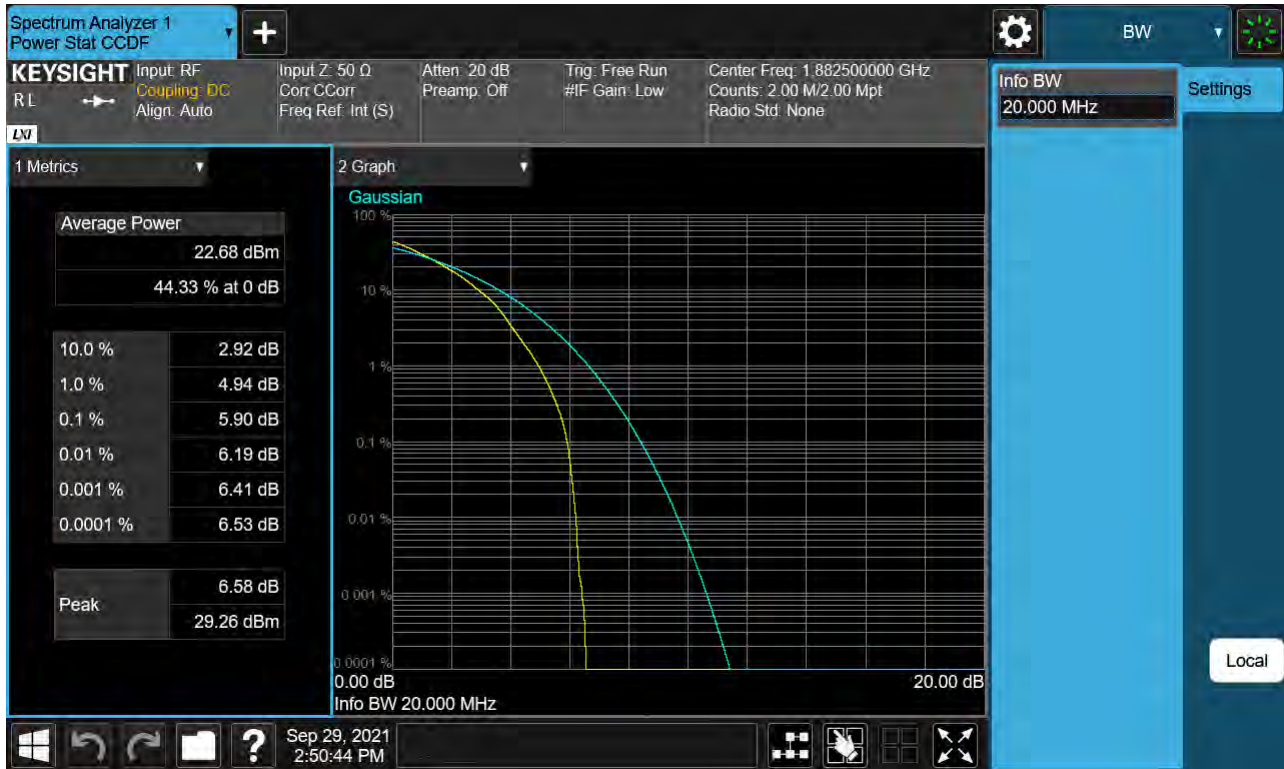
Sub6 n25(2). PAR Plot (20 M BW Ch.376500 64QAM _ Full RB _0)
