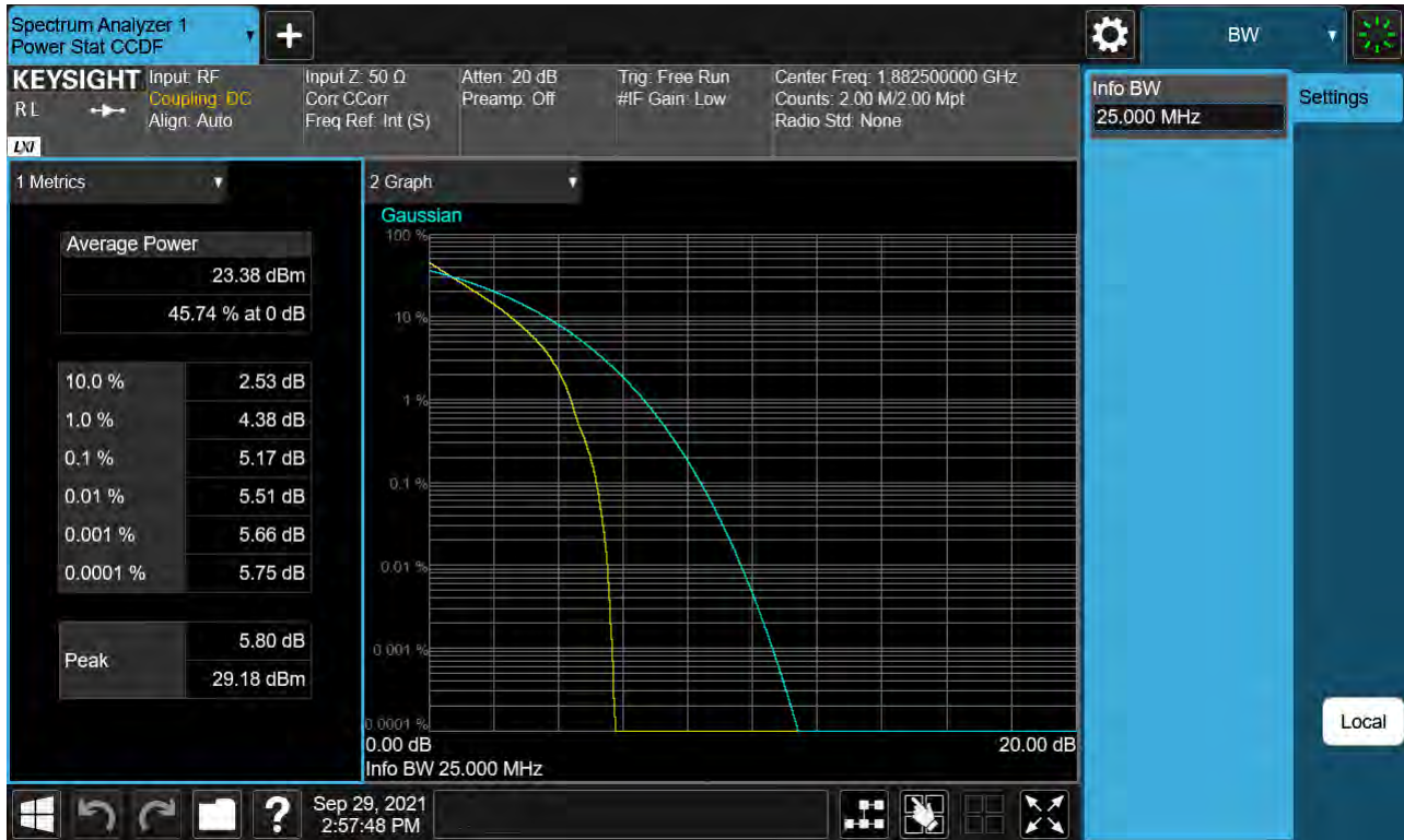
Sub6 n25. PAR Plot (25 M BW Ch.376500 QPSK _ Full RB _0)
