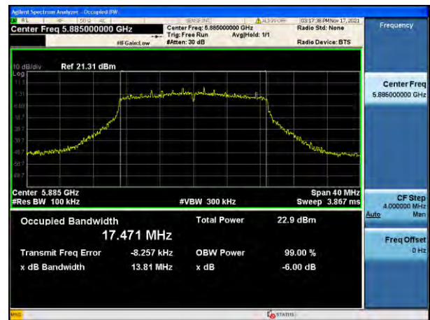
802.11ac(VHT20) (CH.177)
