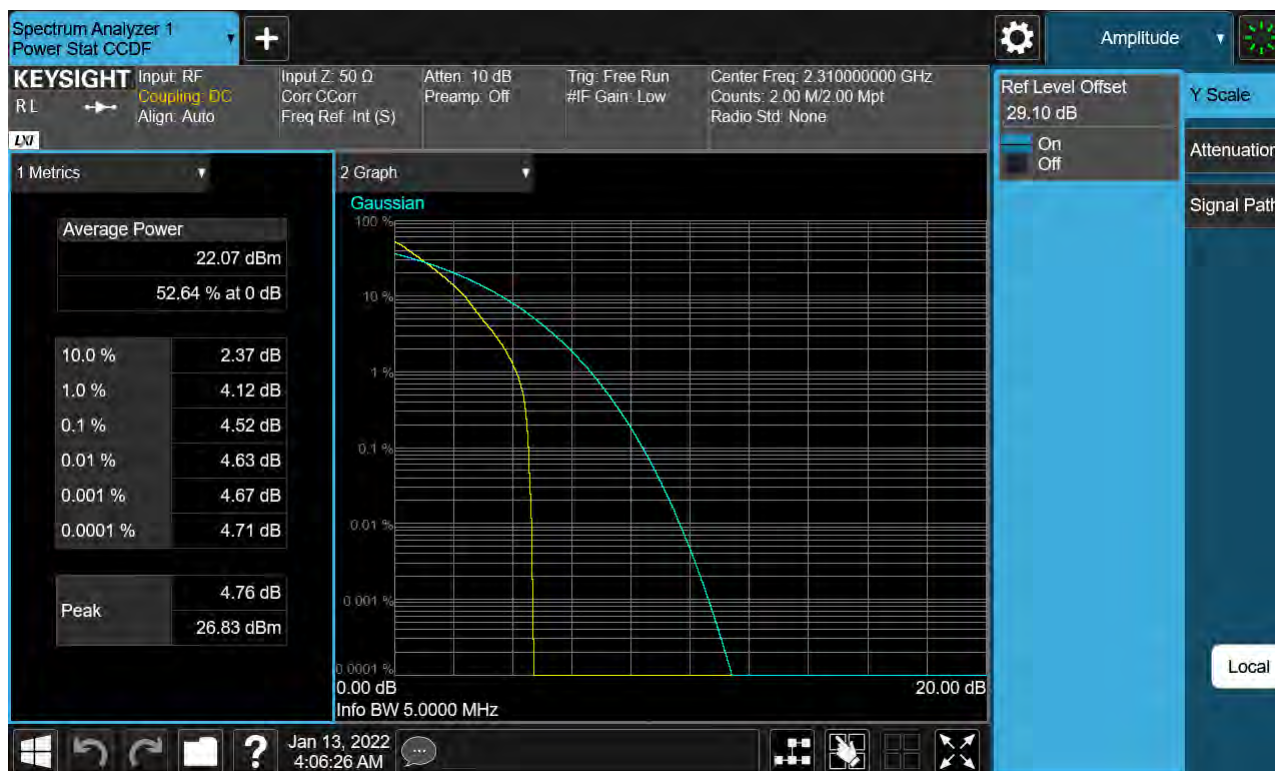
Sub6 n30. PAR Plot (5M BW_Ch.462000_QPSK_RB25_0)
