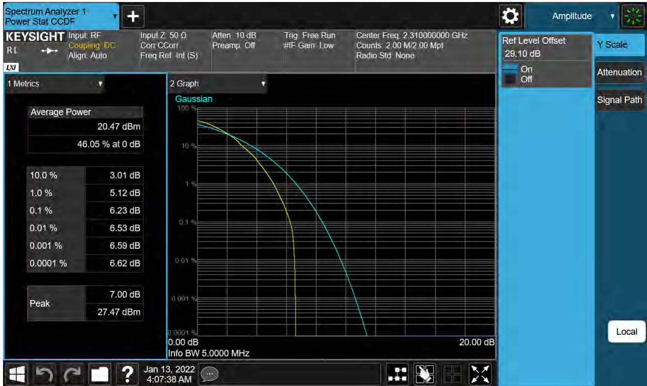
Sub6 n30. PAR Plot (5M BW_Ch.462000_64QAM_RB25_0)
