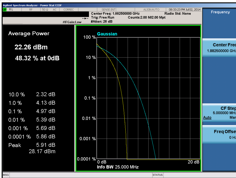
Plot 6-39. PAR Plot (Band 25 – 15.0MHz QPSK – RB Size 75)
