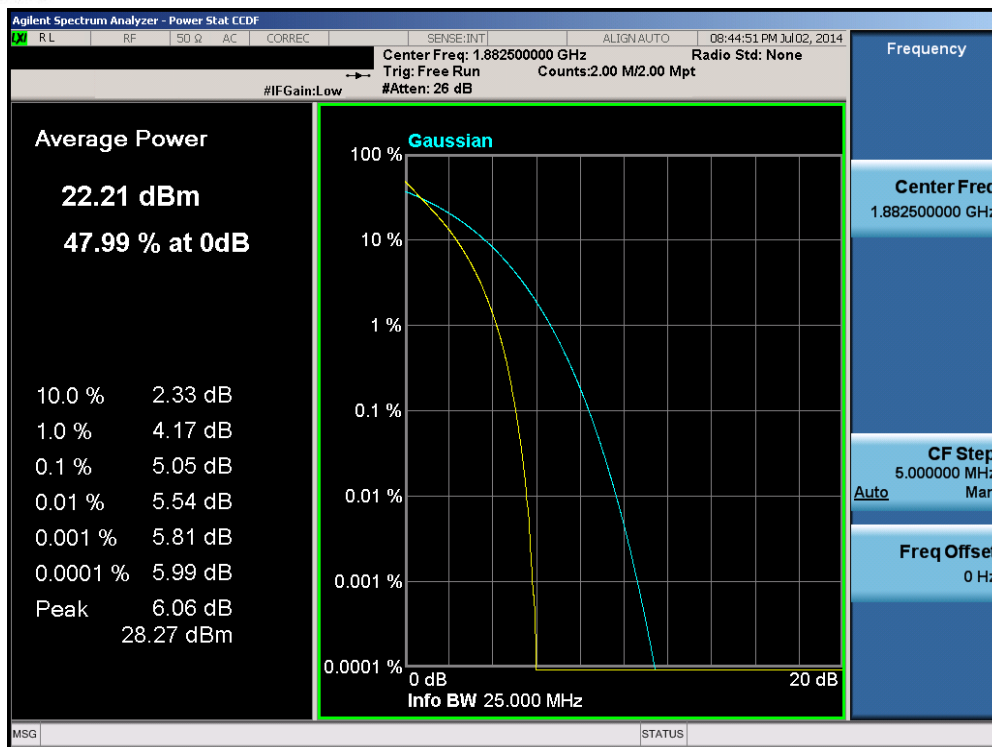
Plot 6-41. PAR Plot (Band 25 – 20.0MHz QPSK – RB Size 100)
