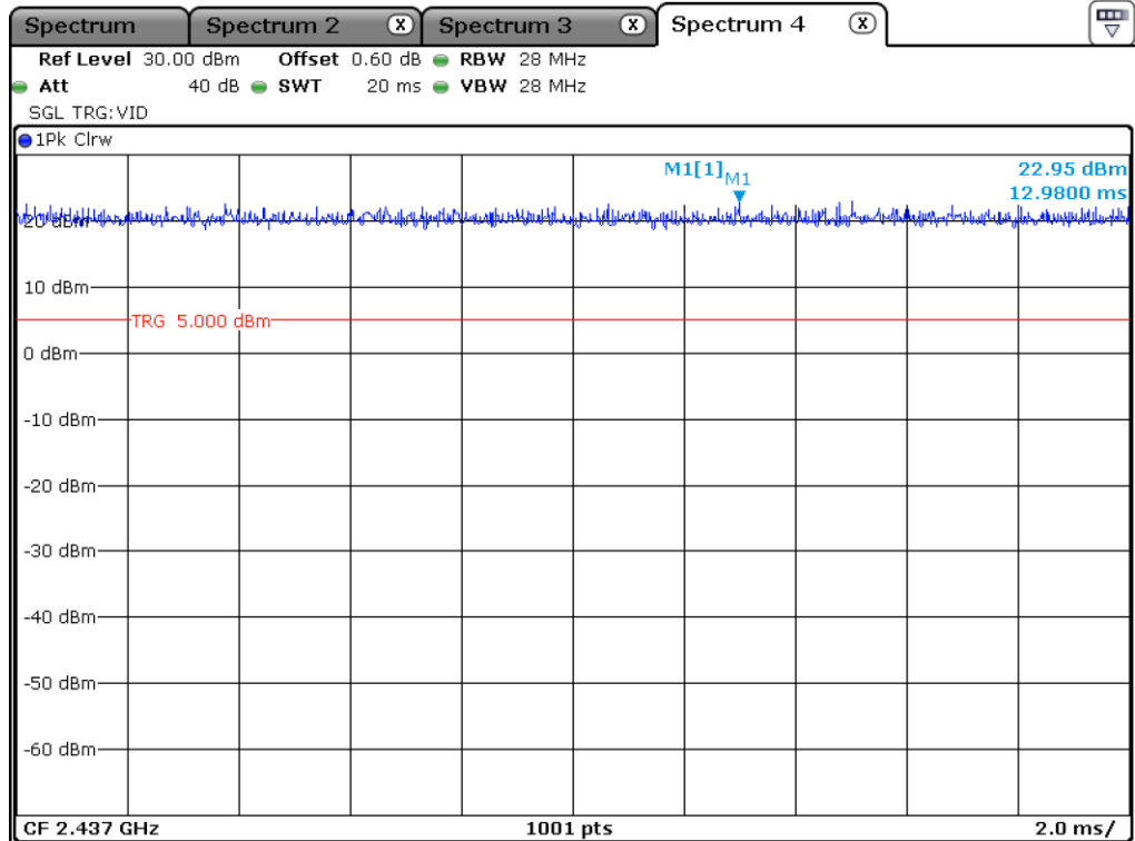
802.11 b_Antenna 1
