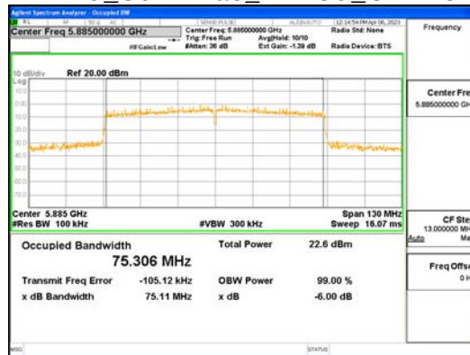
ANT0_802.11ac_VHT80_UNII 4
