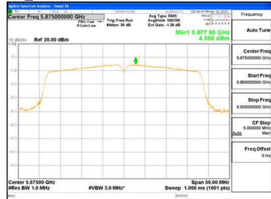
ANTO_802.11n_HT40_UNI1 4
