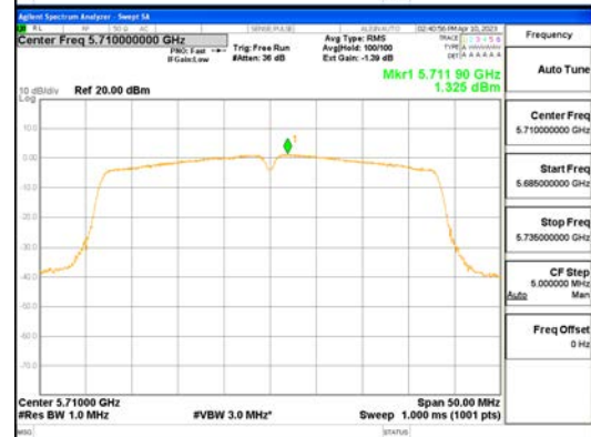
ANTO_802.11n_HT40_UNII 2C
