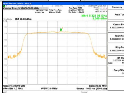
ANT1_802.11ax_HE20_242T_UNII 2A
