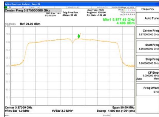
ANTO_802.11ac_VHT40_UNII 4
