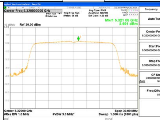
ANT0_802.11ax_HE20_242T_UNII 2A
