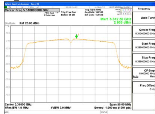
ANTO_802.11n_HT40_UNII 2A
