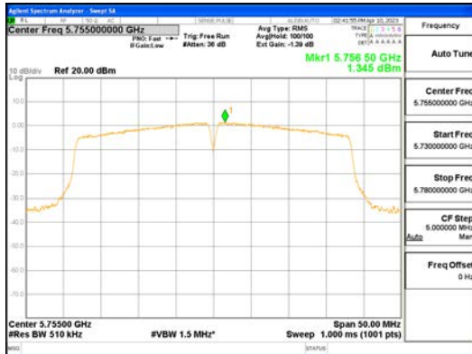
ANTO_802.11n_HT40_UNI1 3
