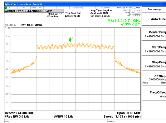
ANT0, 802.11n_HT20
