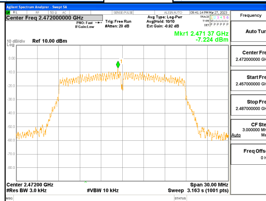
ANT0, 802.11n_HT20
