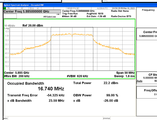
ANT L_802.11a_UNII 4
