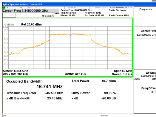
ANT L_802.11a_UNII 4
