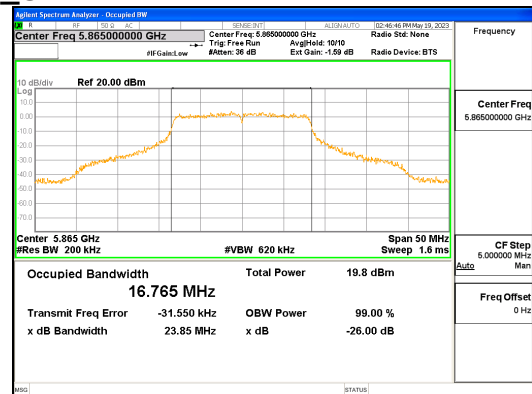
ANT L_802.11a_UNII 4
