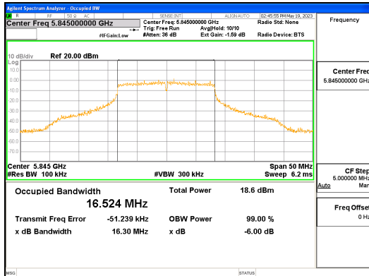
ANT L_802.11a_UNII 4
