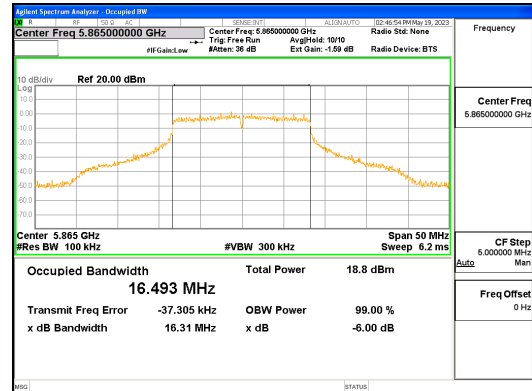
ANT L_802.11a_UNII 4
