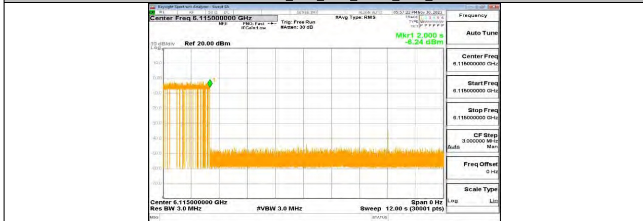
11AX20MIMO_Ant0_6115_Center_6115_5
