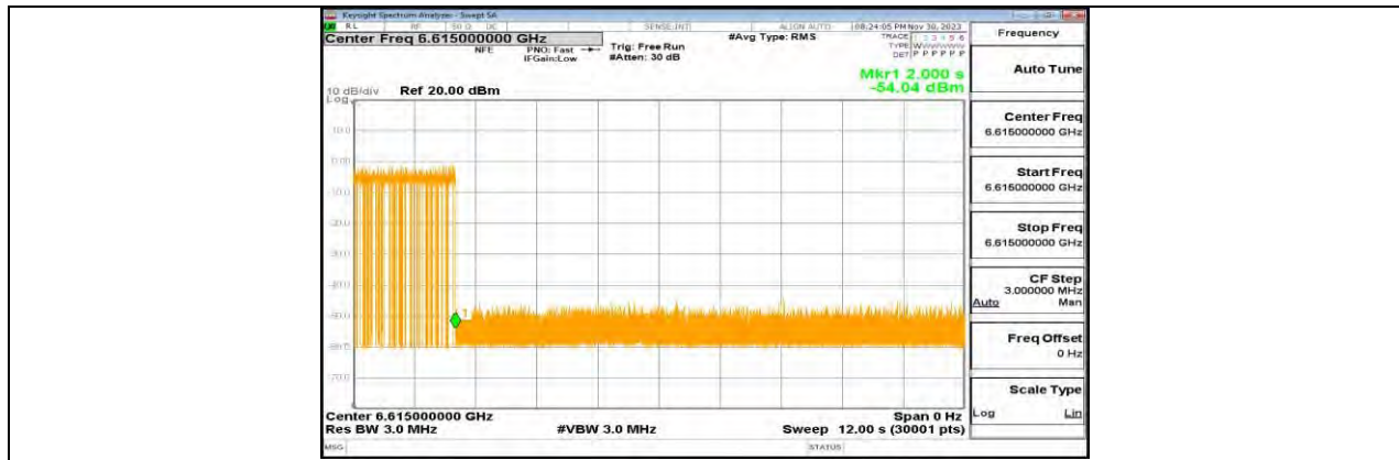
11AX20MIMO_Ant0_6615_Center_6615_5
