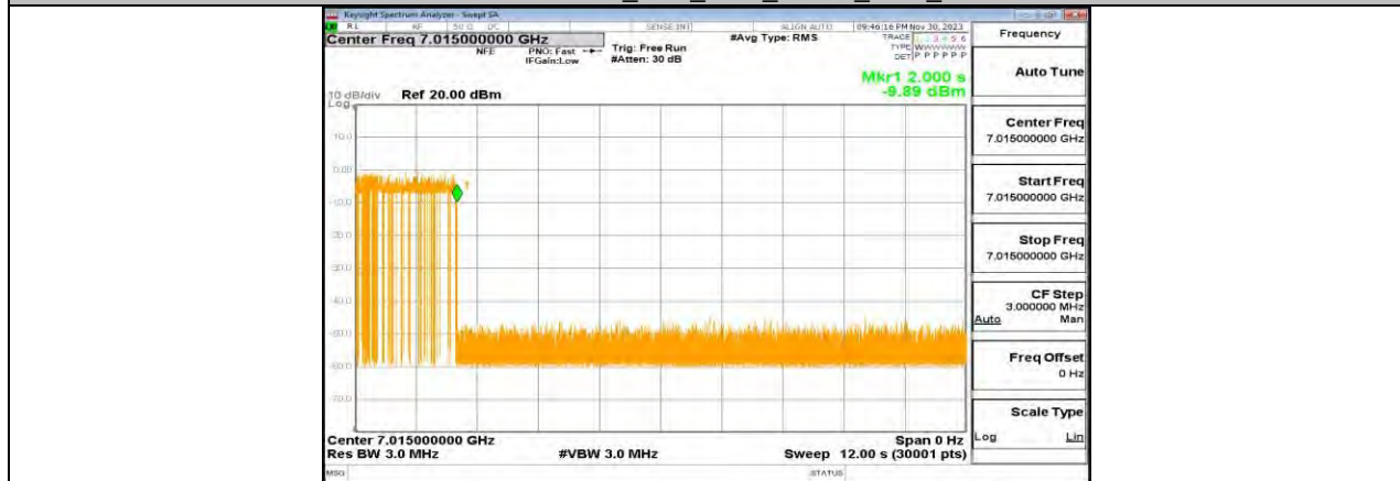
11AX20MIMO_Ant0_7015_Center_7015_5
