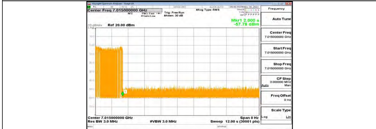
11AX20MIMO_Ant0_7015_Center_7015_2
