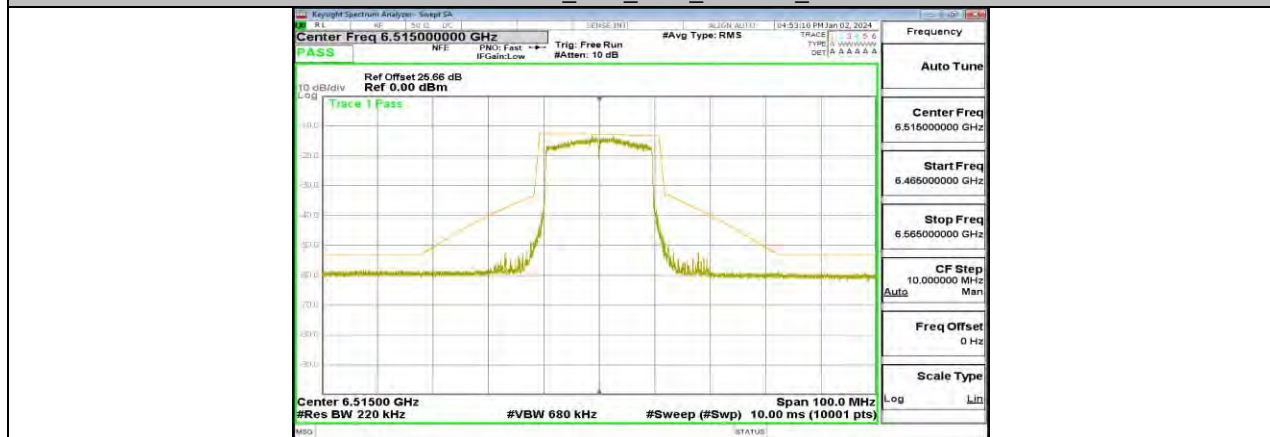
11AX20MIMO_Ant1_6515_242Tone_RU61
