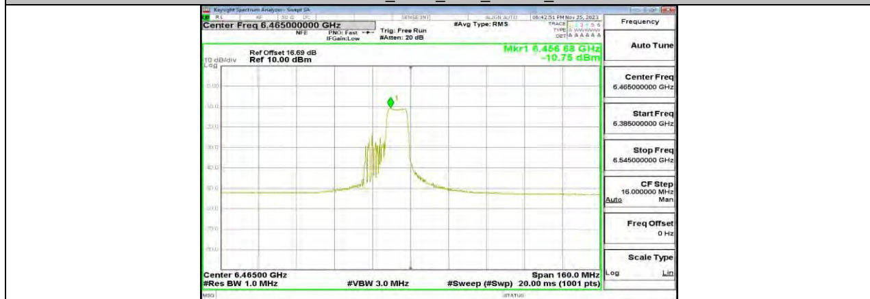
11AX80MIMO_ANT1_6465_106Tone_RU56
