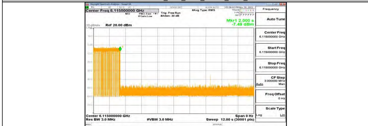
11AX20MIMO_Ant0_6115_Center_6115_6
