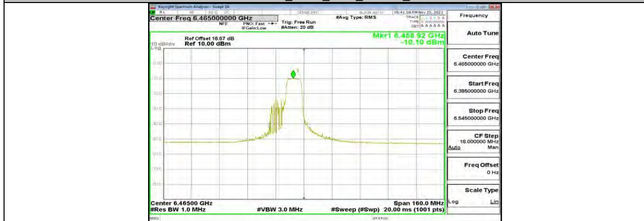
11AX80MIMO_ANT0_6465_52Tone_RU44
