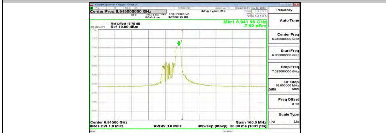
11AX80MIMO_ANT0_6945_26Tone_RU17
