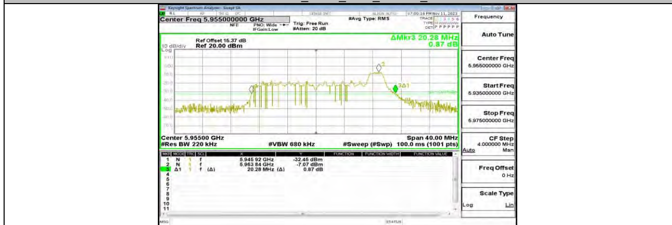
11AX20MIMO_ANT1_5955_26Tone_RU8
