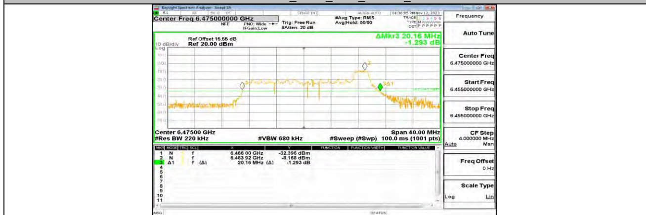
11AX20MIMO_ANT1_6475_26Tone_RU4
