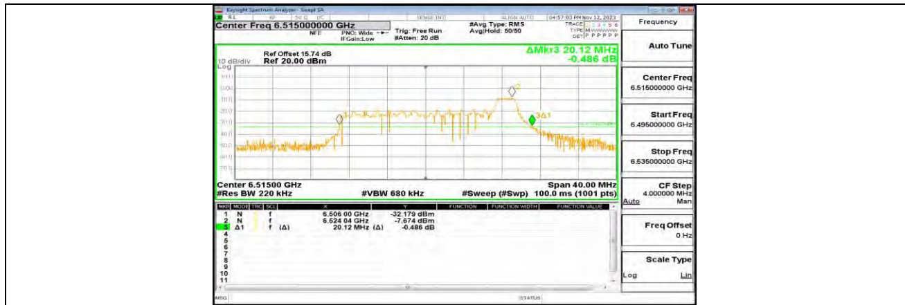
11AX20MIMO_ANT1_6515_26Tone_RU8
