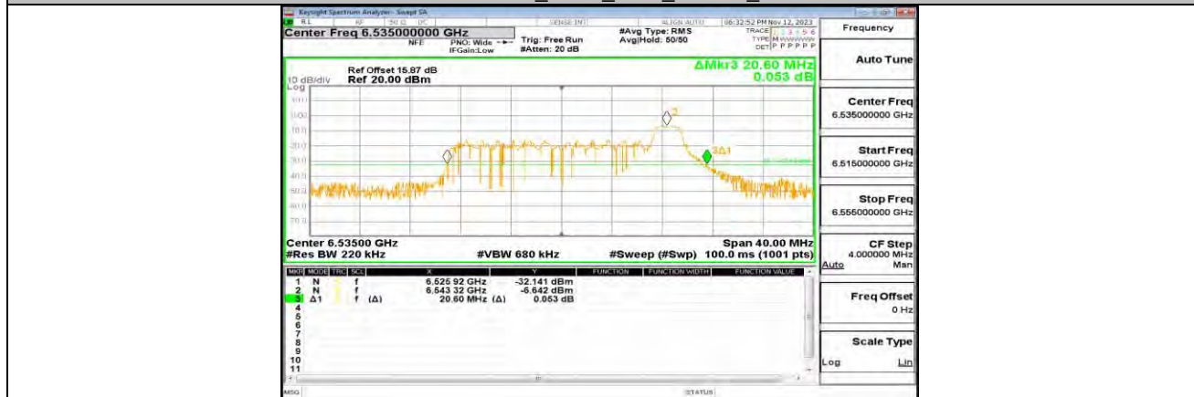
11AX20MIMO_ANT0_6535_26Tone_RU8
