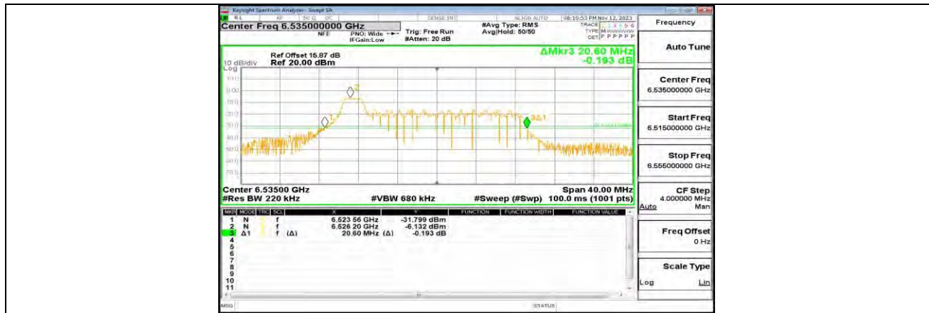
11AX20MIMO_ANT0_6535_26Tone_RU0
