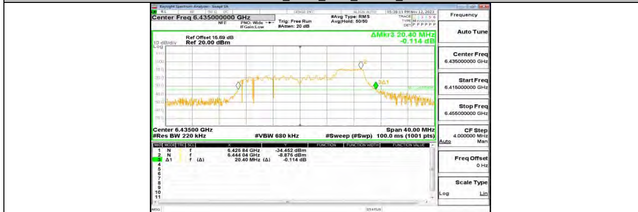
11AX20MIMO_ANT1_6435_52Tone_RU40
