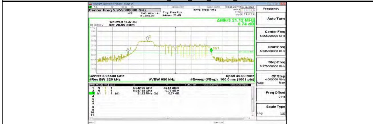
11AX20MIMO_ANT1_5955_52Tone_RU37
