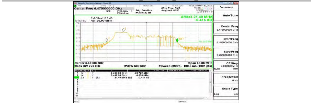
11AX20MIMO_ANT0_6475_52Tone_RU37
