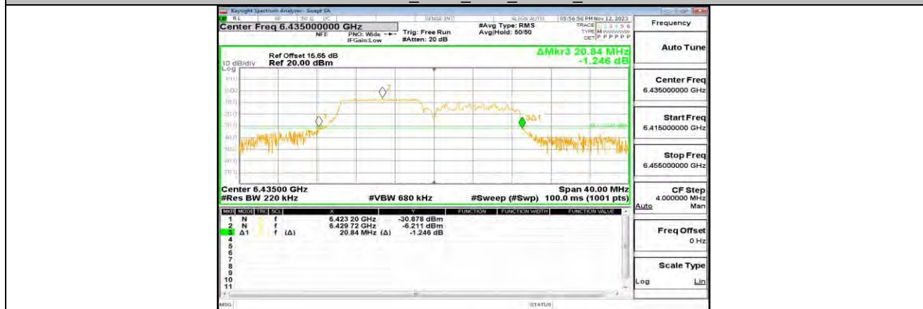
11AX20MIMO_ANT0_6435_106Tone_RU53
