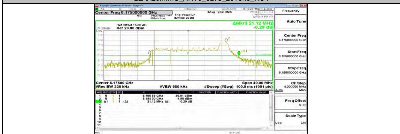
11AX20MIMO_ANT0_6175_26Tone_RU4
