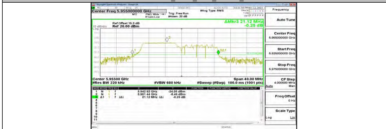
11AX20MIMO_ANT0_5955_52Tone_RU40
