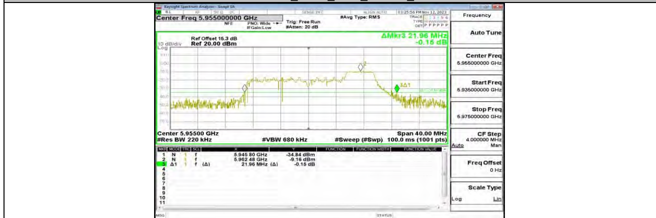
11AX20MIMO_ANT0_5955_52Tone_RU40
