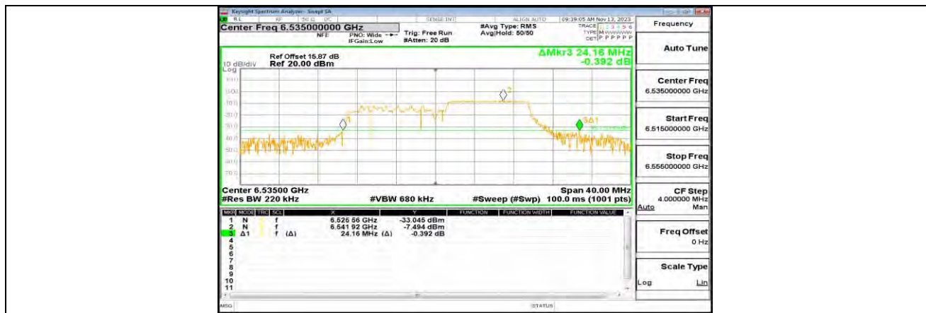
11AX20MIMO_ANT0_6535_106Tone_RU54
