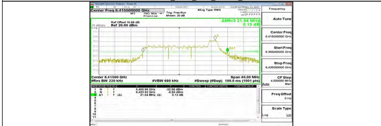
11AX20MIMO_ANT1_6415_26Tone_RU8
