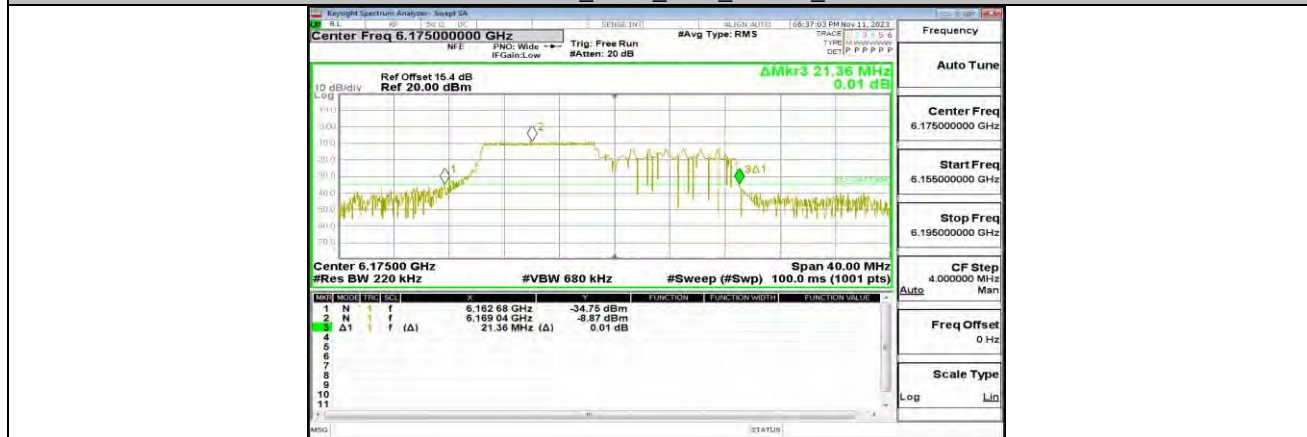
11AX20MIMO_ANT1_6175_106Tone_RU53
