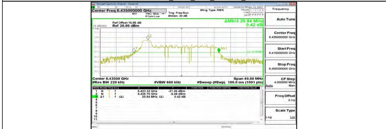
11AX20MIMO_ANT0_6435_26Tone_RU0
