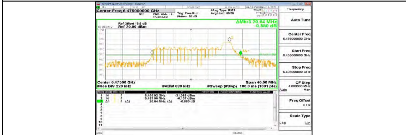
11AX20MIMO_ANT0_6475_26Tone_RU8
