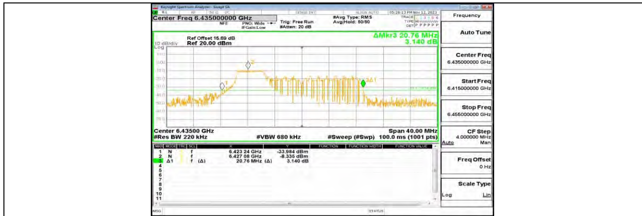
11AX20MIMO_ANT1_6435_52Tone_RU37
