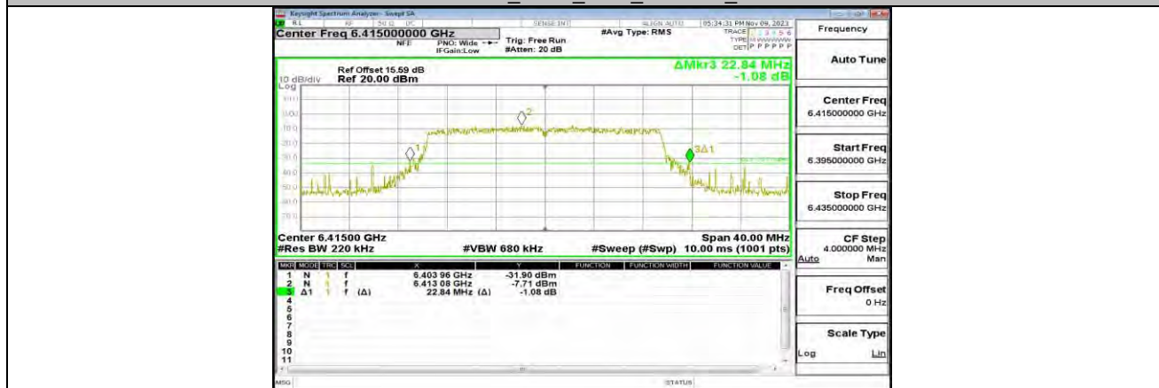
11AX20MIMO_ANT1_6415_242Tone_RU61
