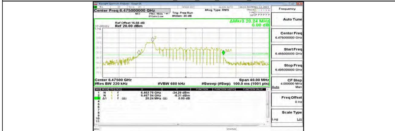
11AX20MIMO_ANT1_6475_26Tone_RU0
