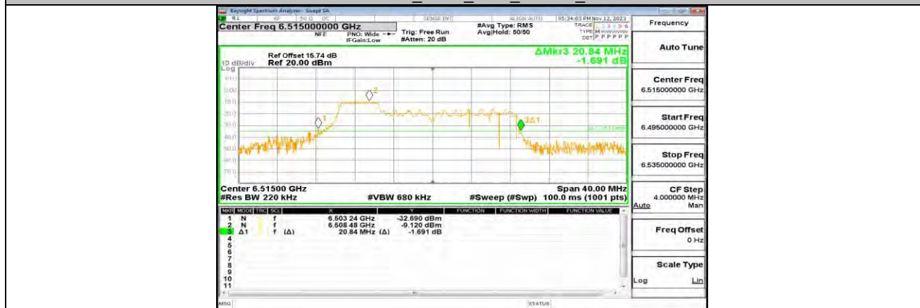
11AX20MIMO_ANT1_6515_52Tone_RU37
