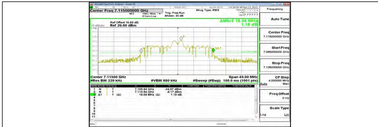
11AX20MIMO_ANT0_7115_26Tone_RU4
