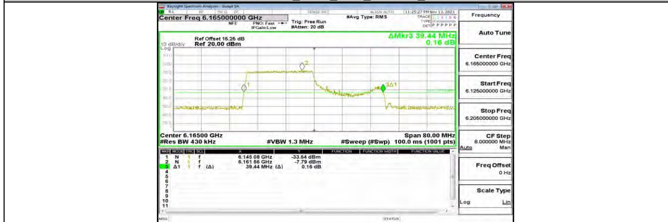
11AX40MIMO_ANT0_6165_242Tone_RU61
