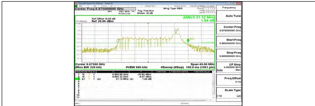
11AX20MIMO_ANT0_6875_26Tone_RU8
