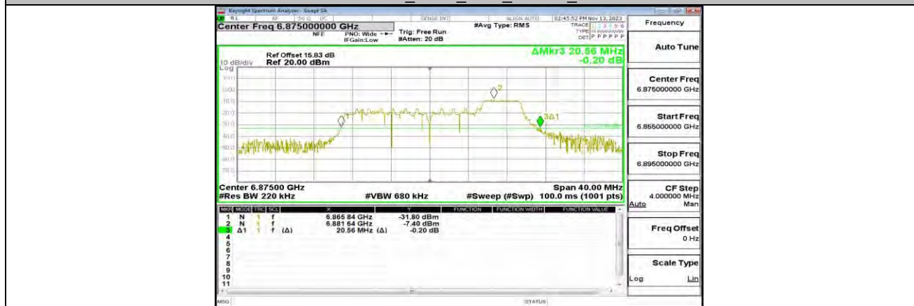
11AX20MIMO_ANT0_6875_52Tone_RU38
