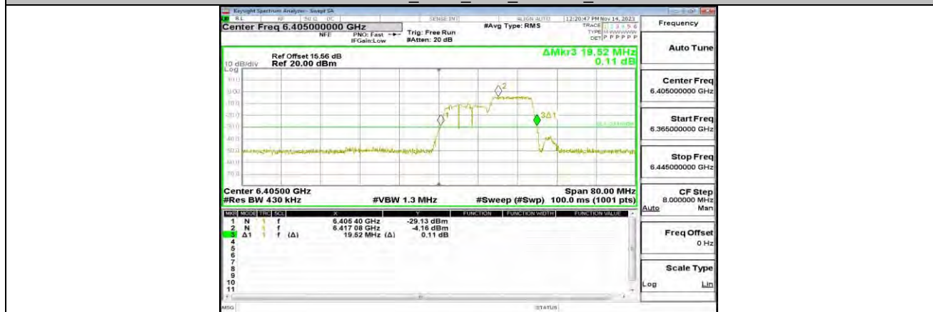
11AX40MIMO_ANT0_6405_106Tone_RU54
