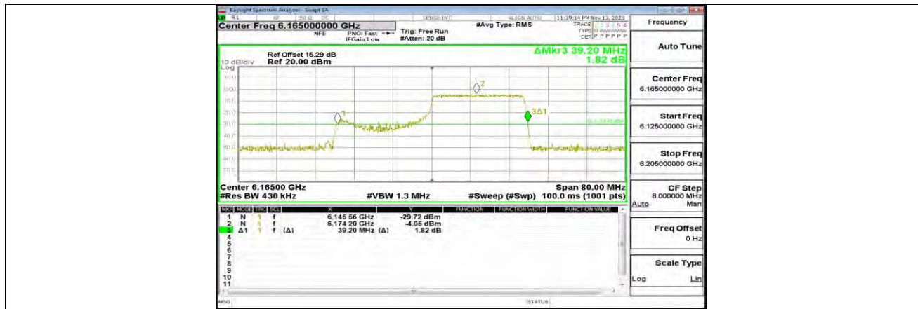
11AX40MIMO_ANT1_6165_242Tone_RU62
