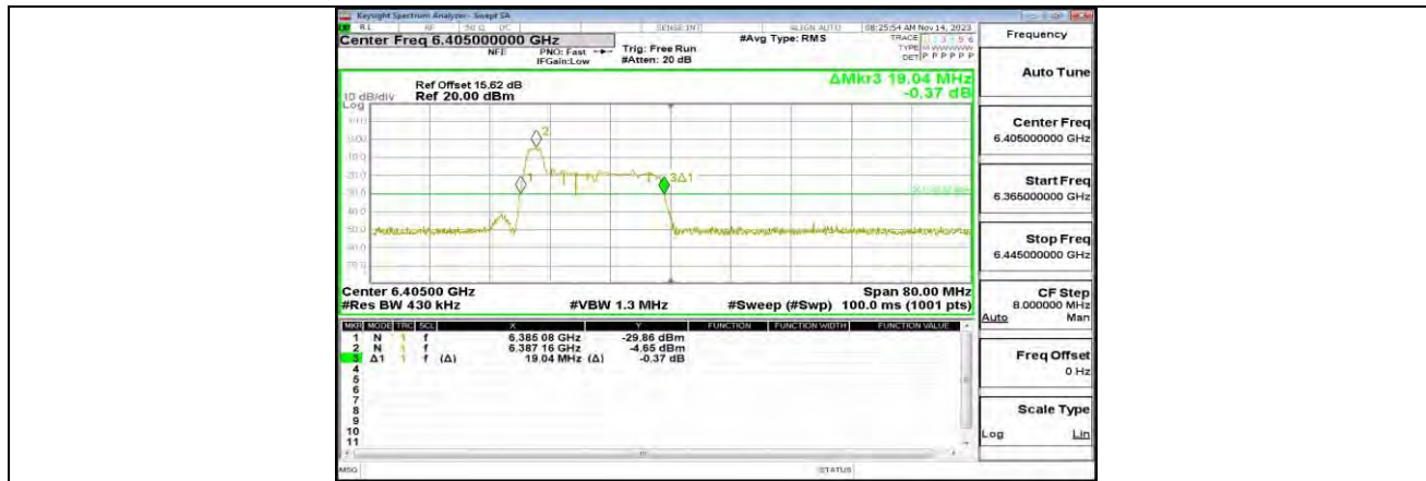
11AX40MIMO_ANT1_6405_26Tone_RU0
