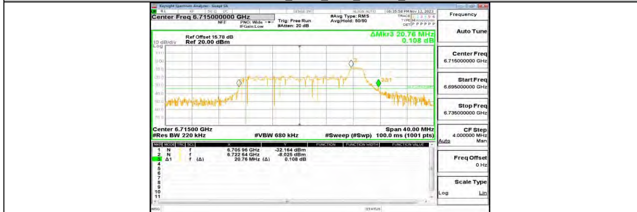
11AX20MIMO_ANT1_6715_26Tone_RU8
