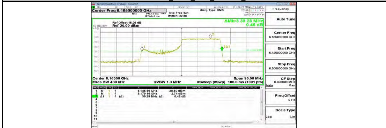
11AX40MIMO_ANT0_6165_242Tone_RU62
