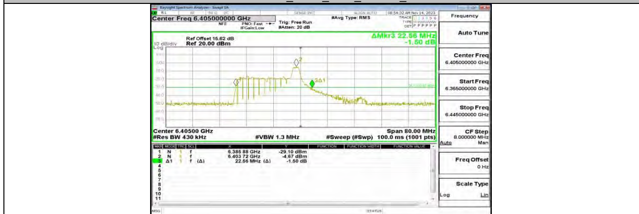
11AX40MIMO_ANT1_6405_26Tone_RU8
