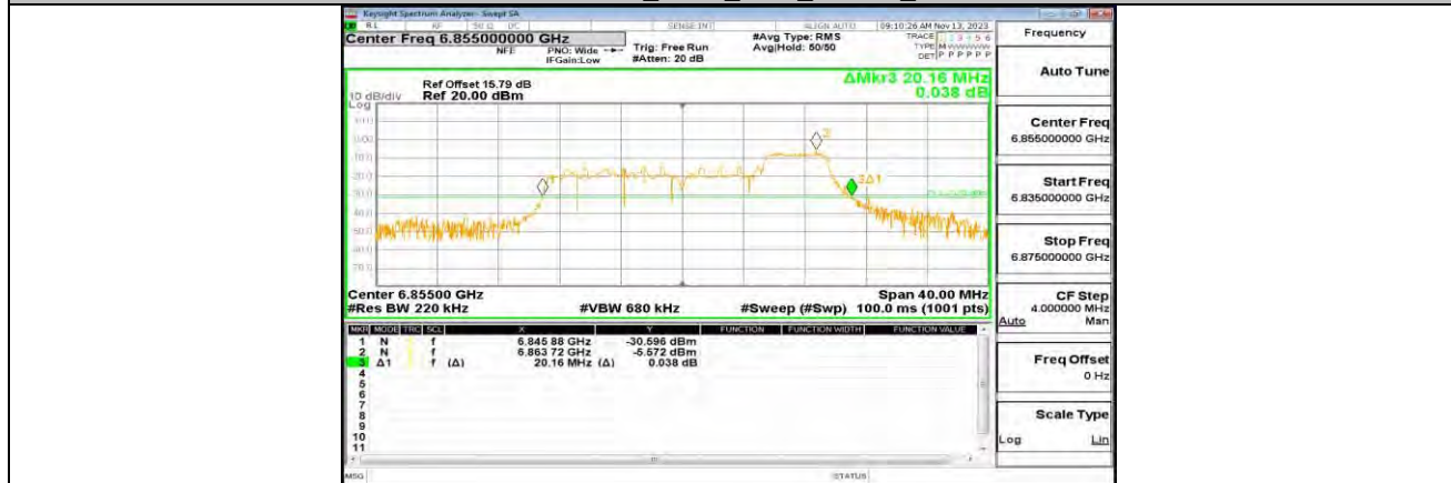
11AX20MIMO_ANT1_6855_52Tone_RU40
