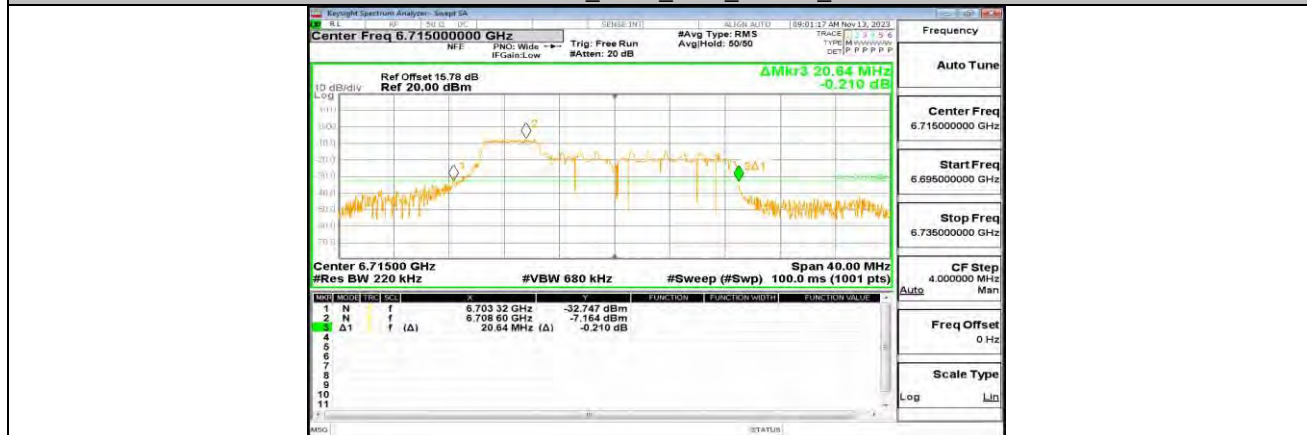
11AX20MIMO_ANT1_6715_52Tone_RU37
