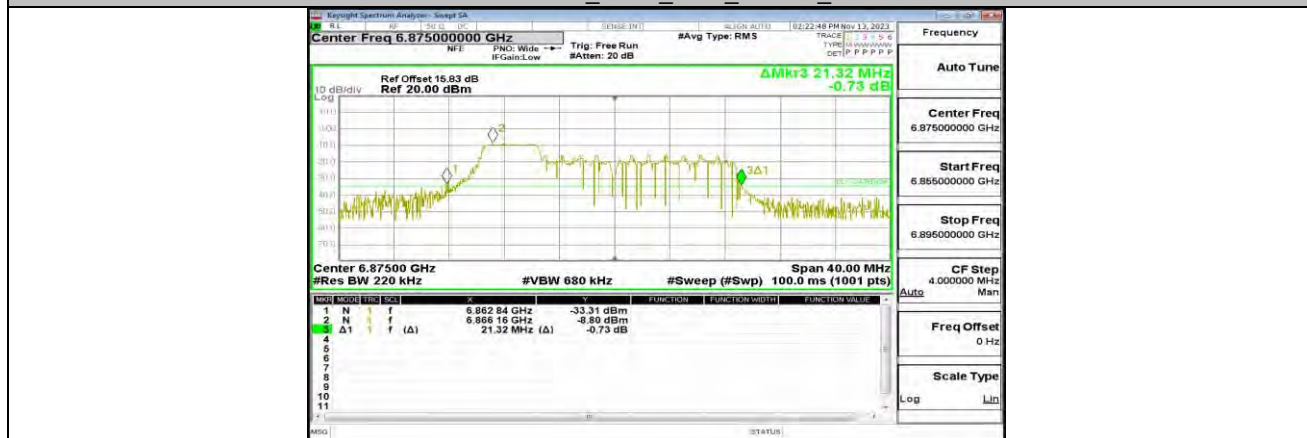
11AX20MIMO_ANT0_6875_52Tone_RU37
