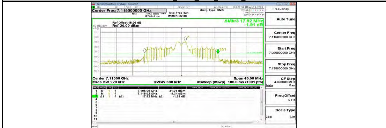
11AX20MIMO_ANT1_7115_26Tone_RU4
