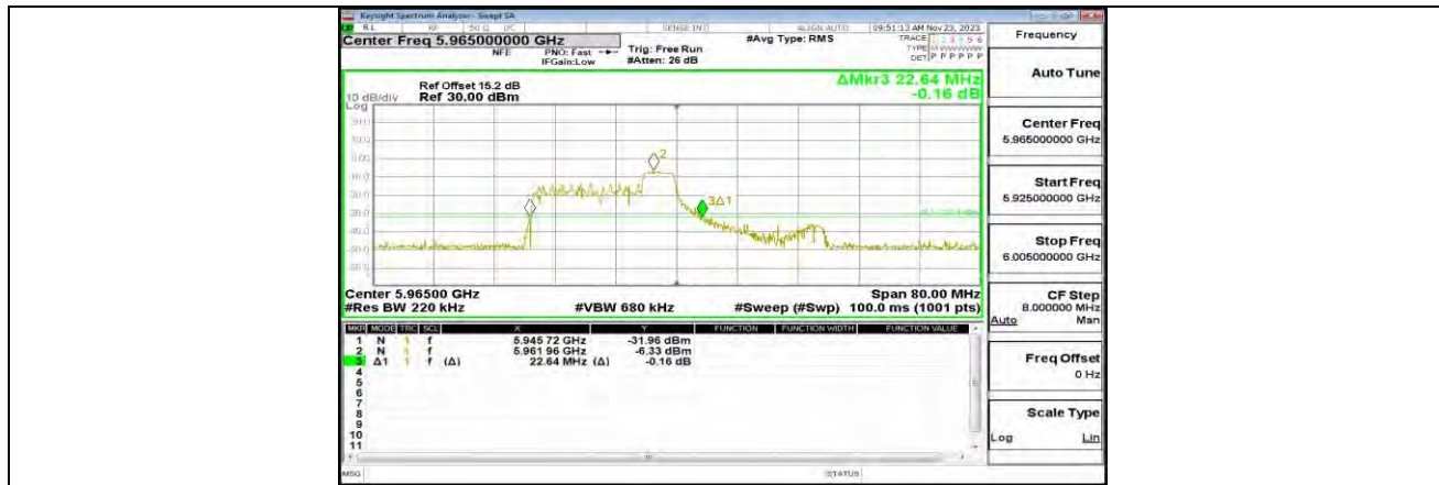
11AX40MIMO_ANT0_5965_52Tone_RU40
