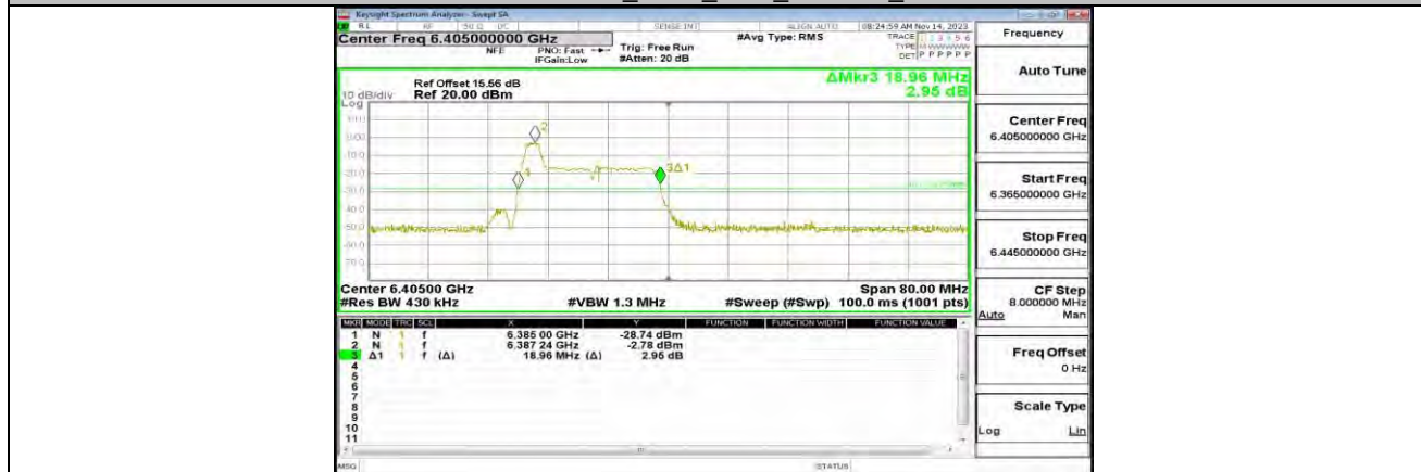
11AX40MIMO_ANT0_6405_26Tone_RU0
