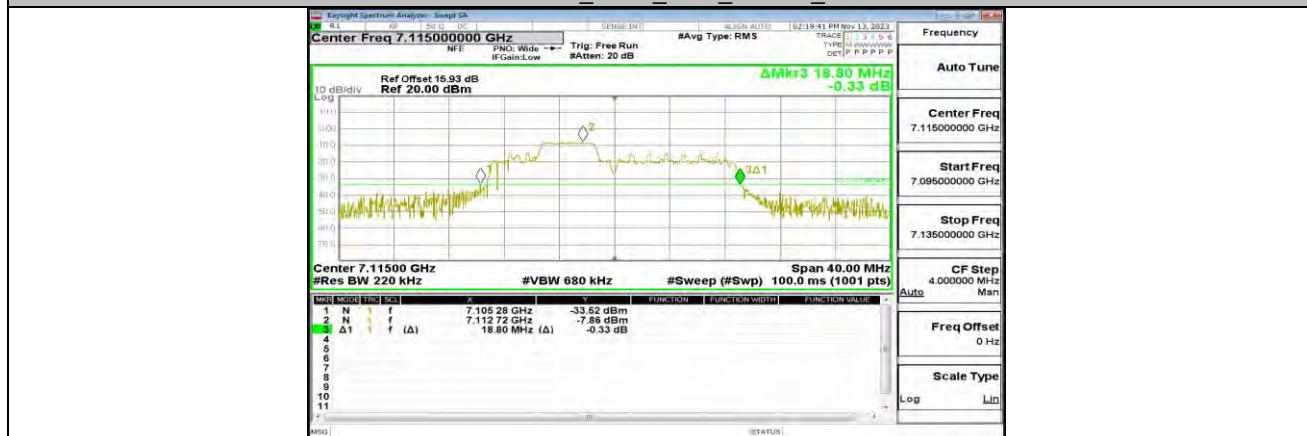
11AX20MIMO_ANT0_7115_52Tone_RU37
