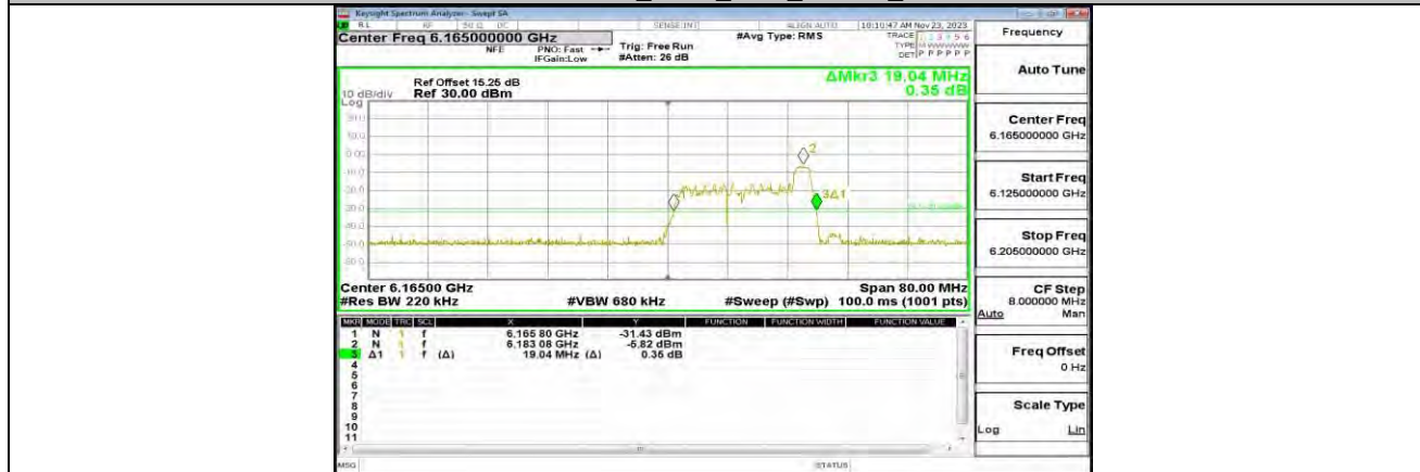
11AX40MIMO_ANT0_6165_26Tone_RU17
