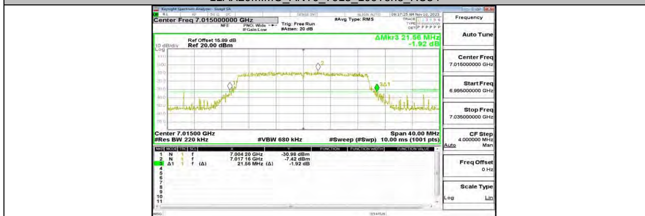
11AX20MIMO_ANT0_7015_106Tone_RU54
