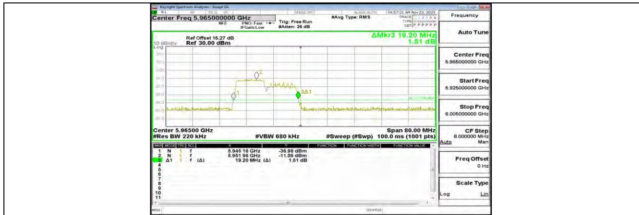
11AX40MIMO_ANT1_5965_106Tone_RU53
