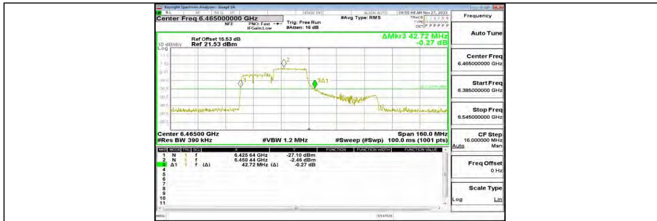
11AX80MIMO_ANT1_6465_242Tone_RU62
