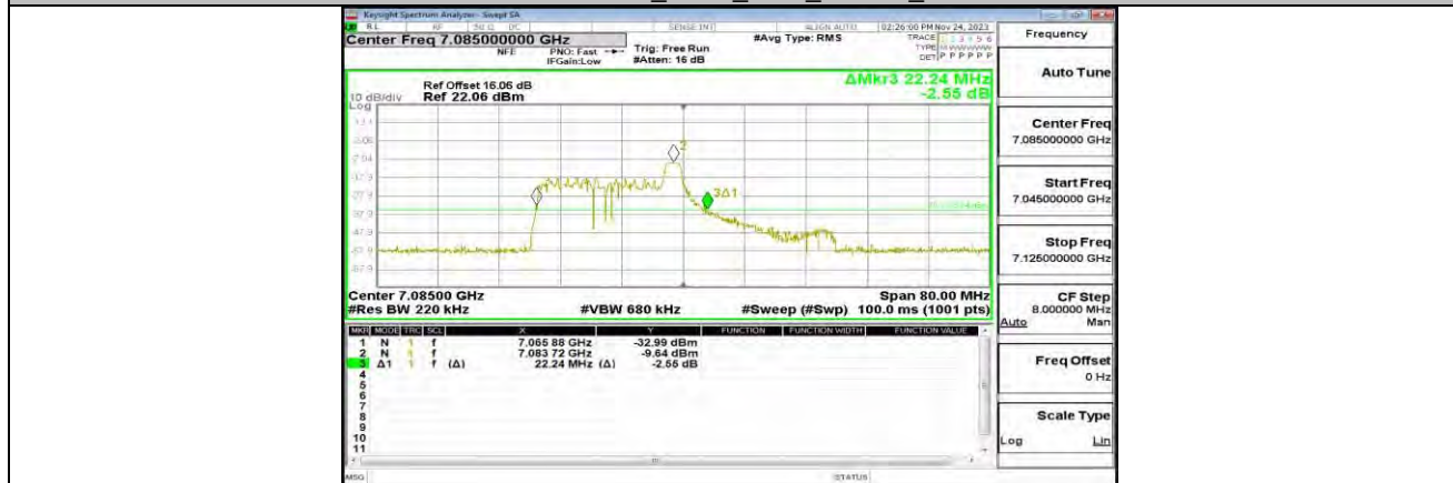
11AX40MIMO_ANT0_7085_26Tone_RU8
