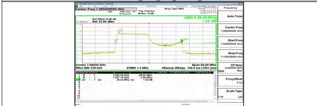
11AX40MIMO_ANT0_7085_106Tone_RU56
