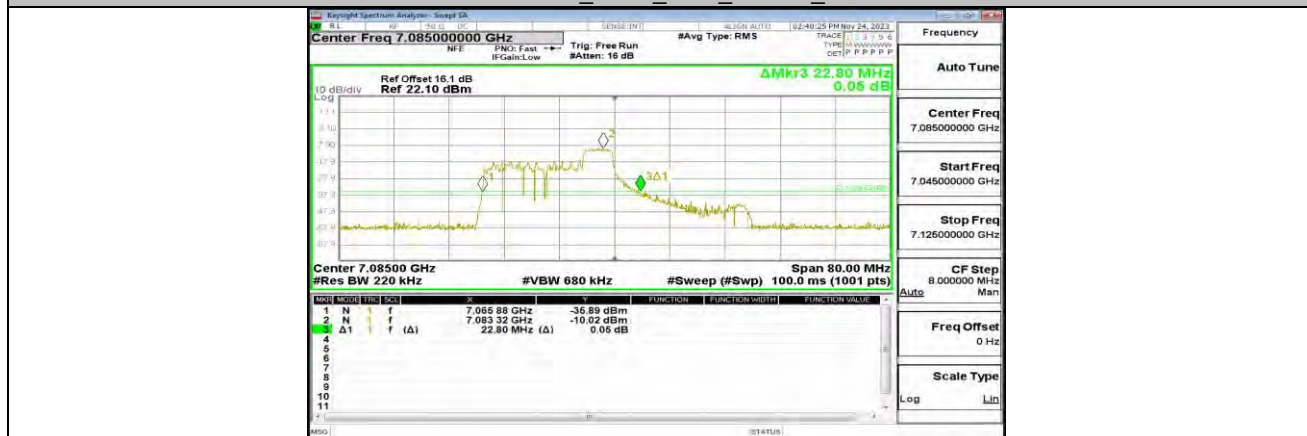
11AX40MIMO_ANT1_7085_52Tone_RU37
