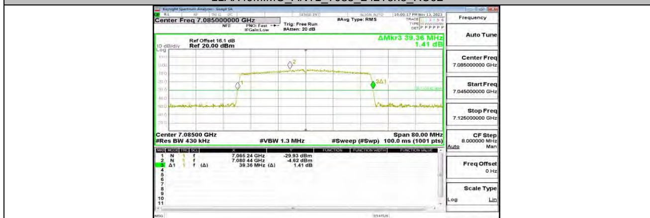
11AX40MIMO_ANT1_7085_242Tone_RU62
