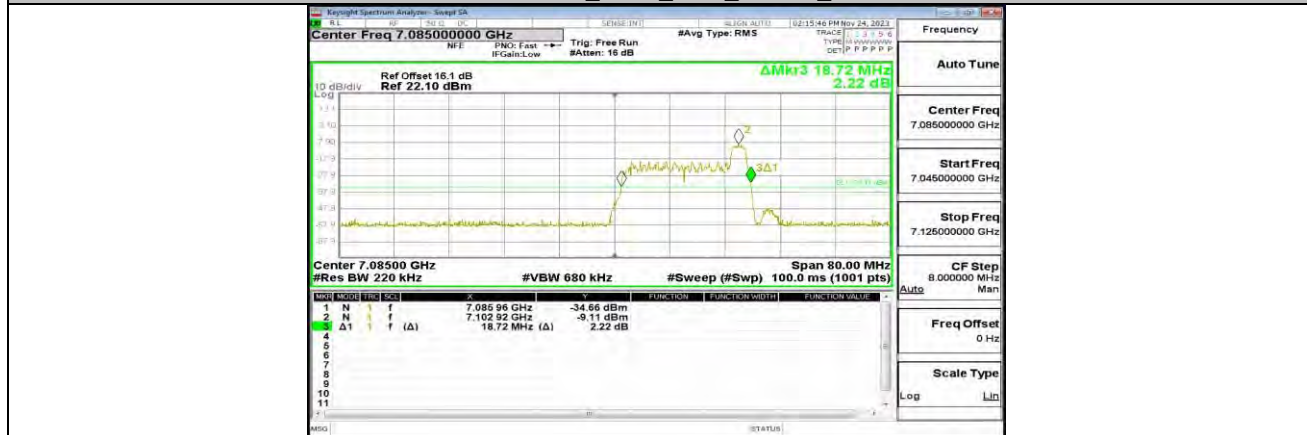
11AX40MIMO_ANT1_7085_26Tone_RU17
