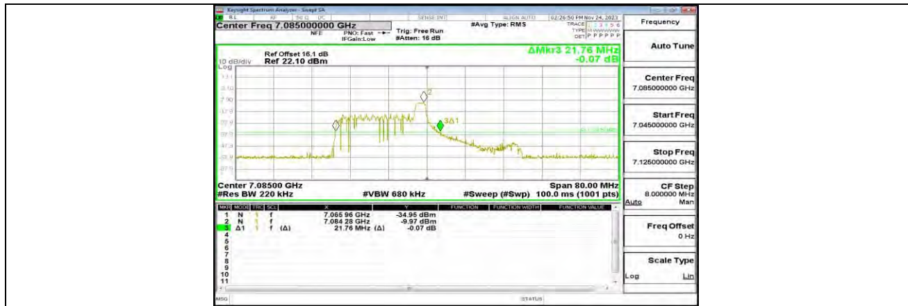
11AX40MIMO_ANT1_7085_26Tone_RU8
