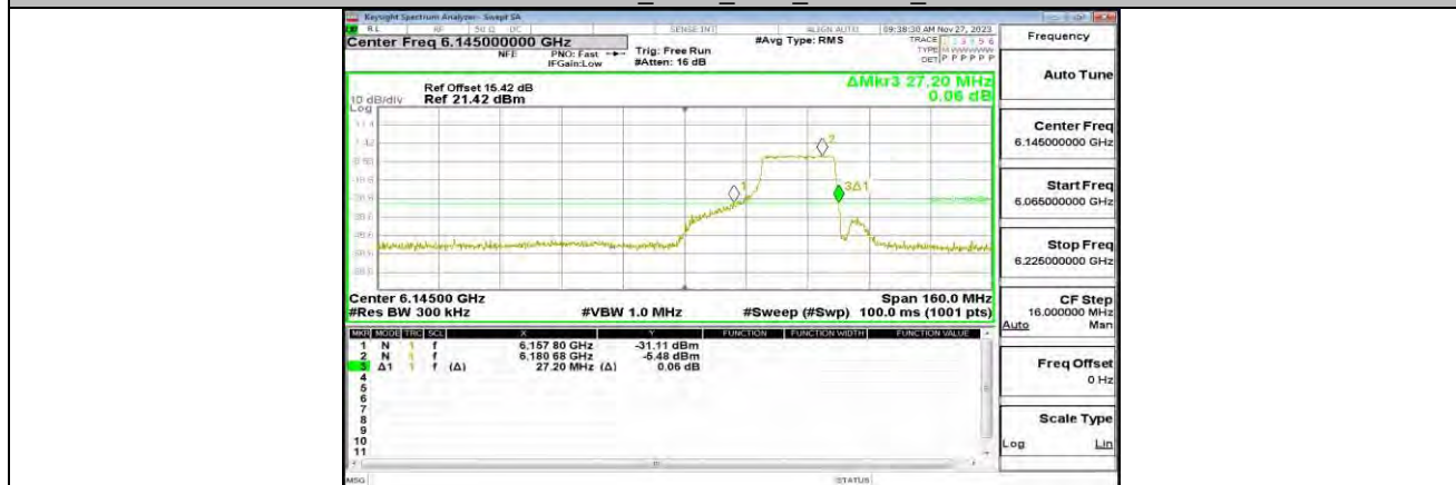
11AX80MIMO_ANT0_6145_242Tone_RU62
