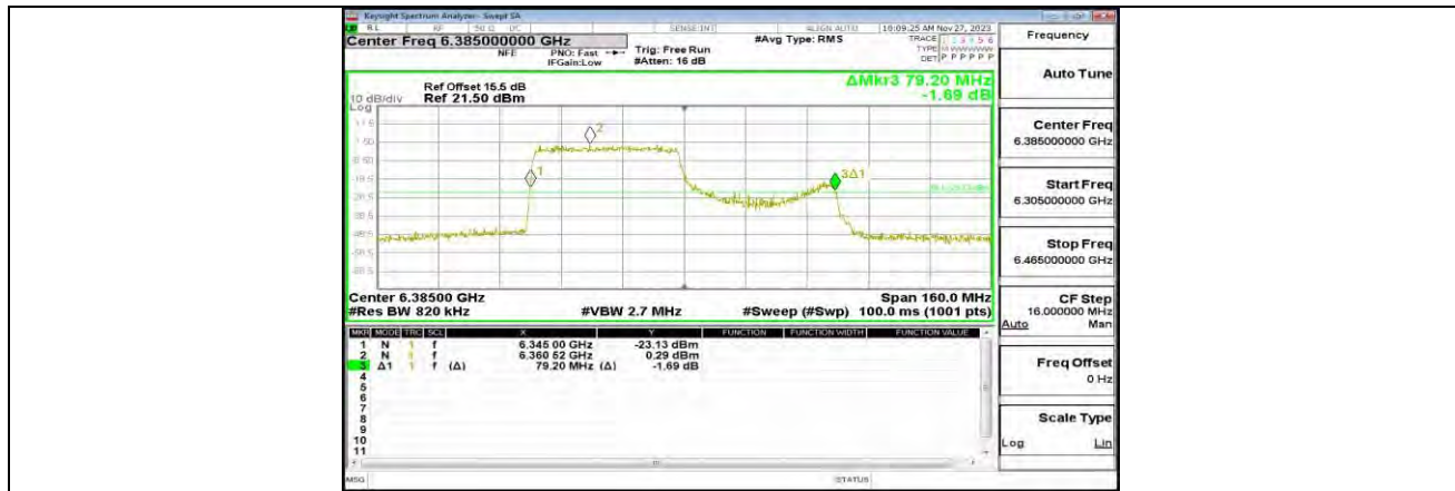
11AX80MIMO_ANT1_6385_484Tone_RU65
