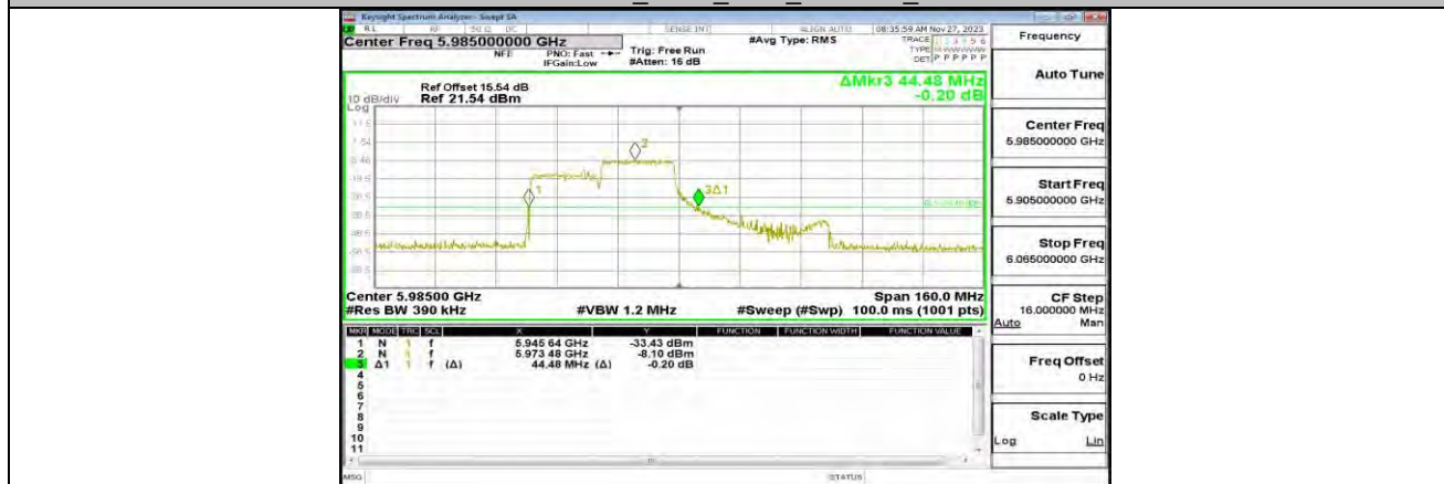
11AX80MIMO_ANT1_5985_242Tone_RU62
