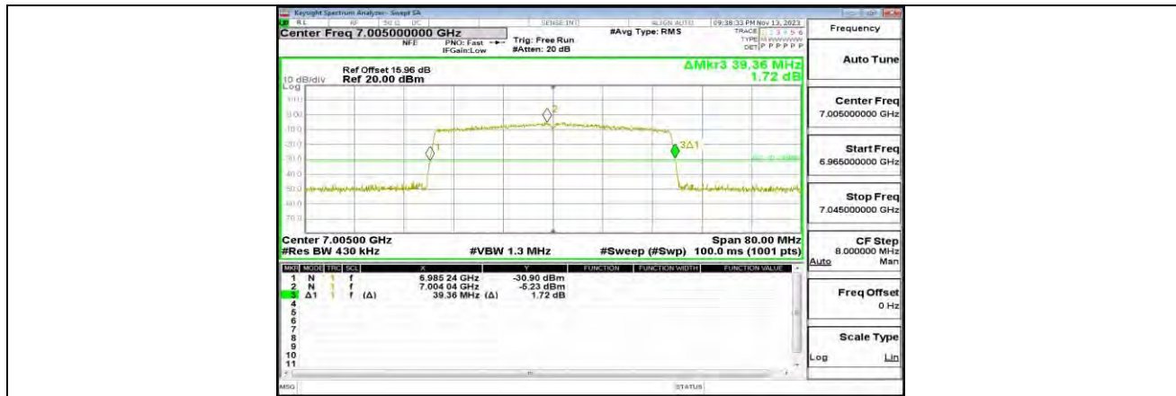
11AX40MIMO_ANT1_7005_484Tone_RU65
