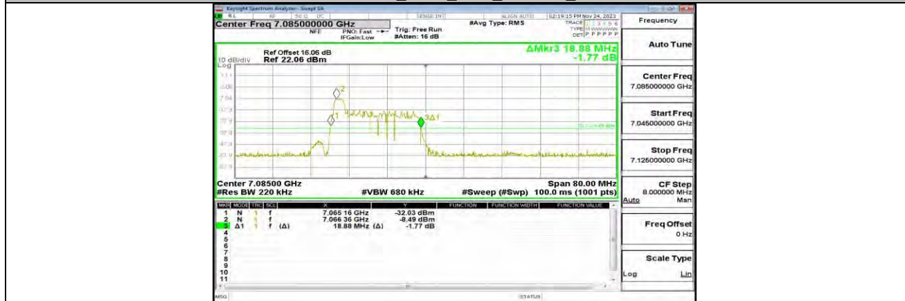
11AX40MIMO_ANT0_7085_26Tone_RU0
