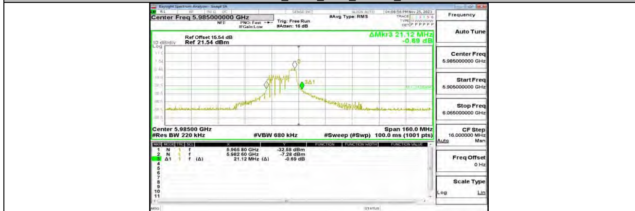
11AX80MIMO_ANT1_5985_52Tone_RU44
