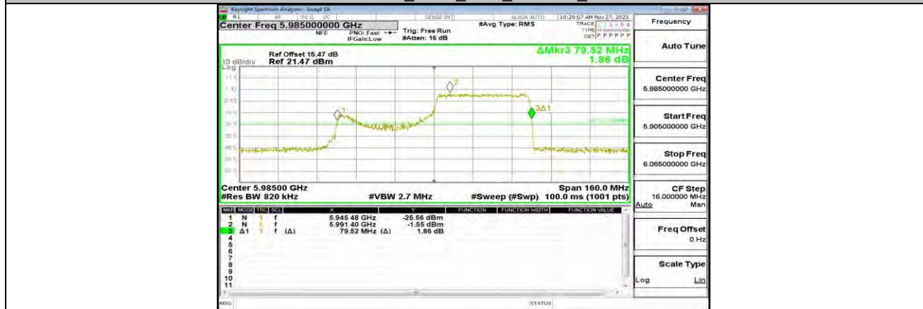
11AX80MIMO_ANT0_5985_484Tone_RU65
