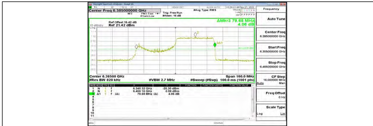
11AX80MIMO_ANT0_6385_484Tone_RU66
