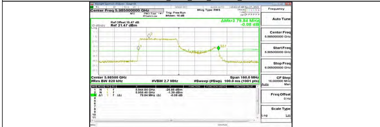
11AX80MIMO_ANT0_5985_484Tone_RU65
