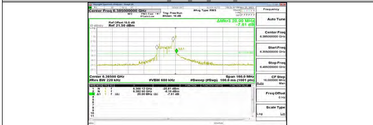
11AX80MIMO_ANT1_6385_26Tone_RU0
