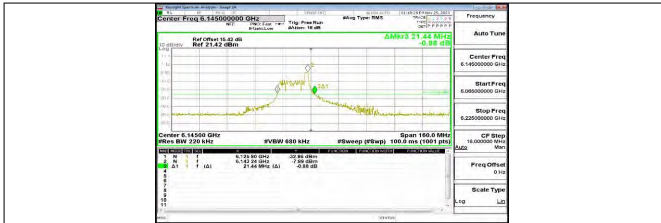
11AX80MIMO_ANT0_6145_26Tone_RU17
