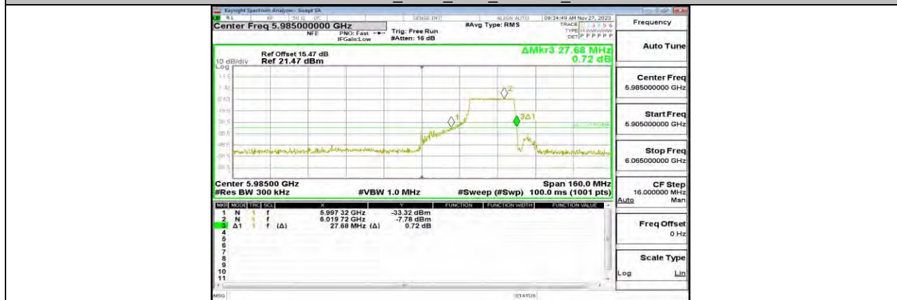
11AX80MIMO_ANT0_5985_242Tone_RU64
