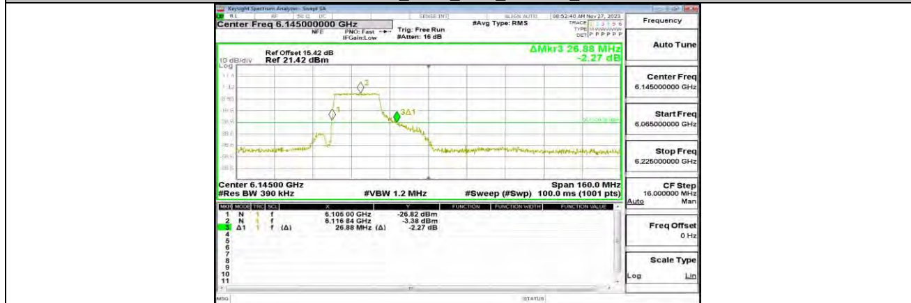
11AX80MIMO_ANT0_6145_242Tone_RU61
