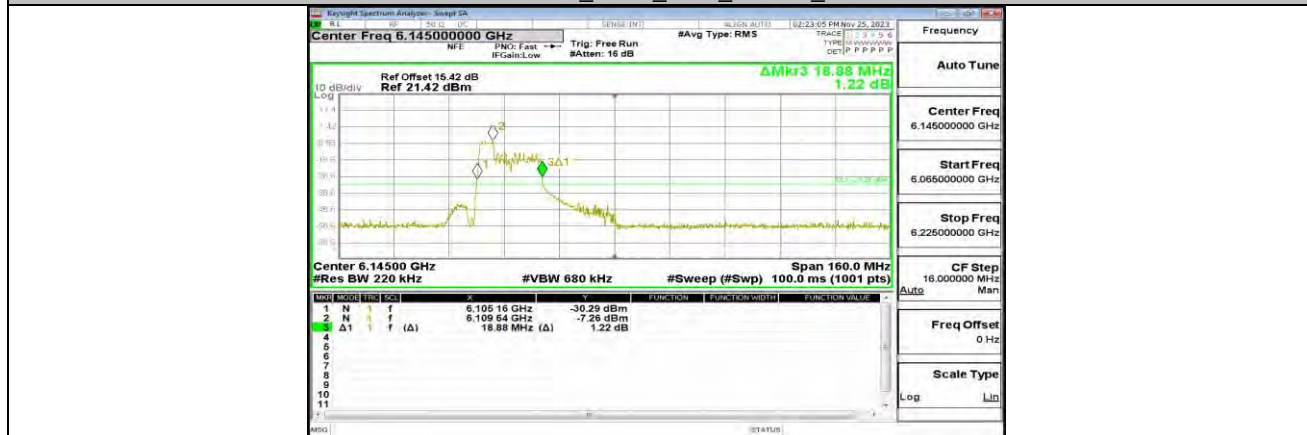
11AX80MIMO_ANT0_6145_52Tone_RU37
