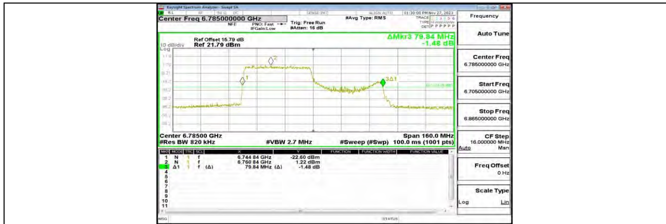
11AX80MIMO_ANT0_6785_484Tone_RU65
