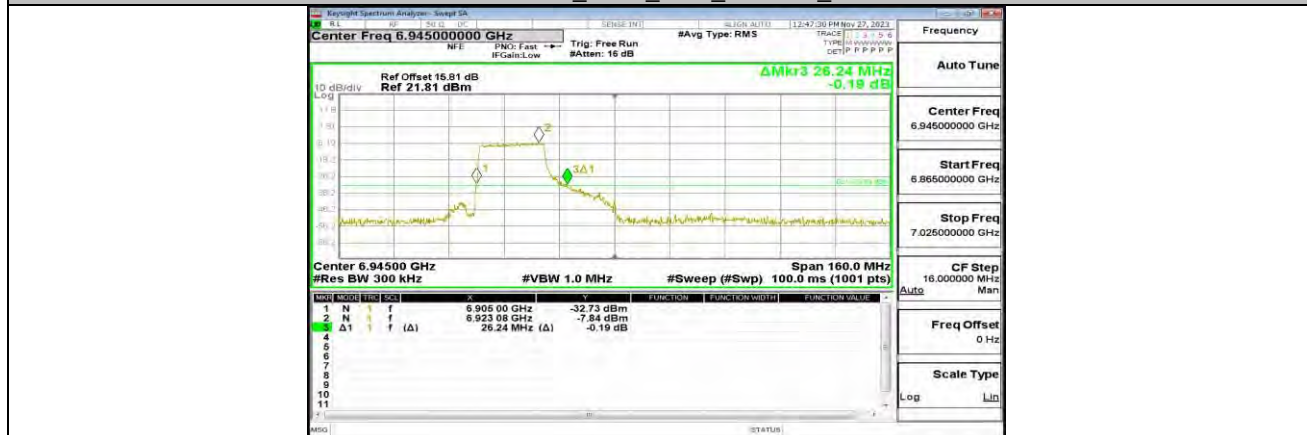
11AX80MIMO_ANT1_6945_242Tone_RU61
