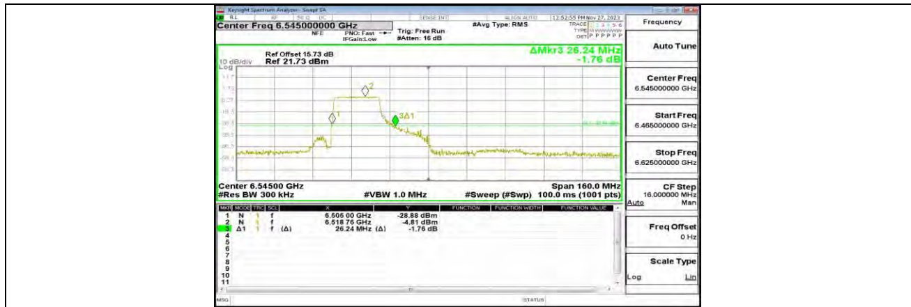
11AX80MIMO_ANT0_6545_242Tone_RU61
