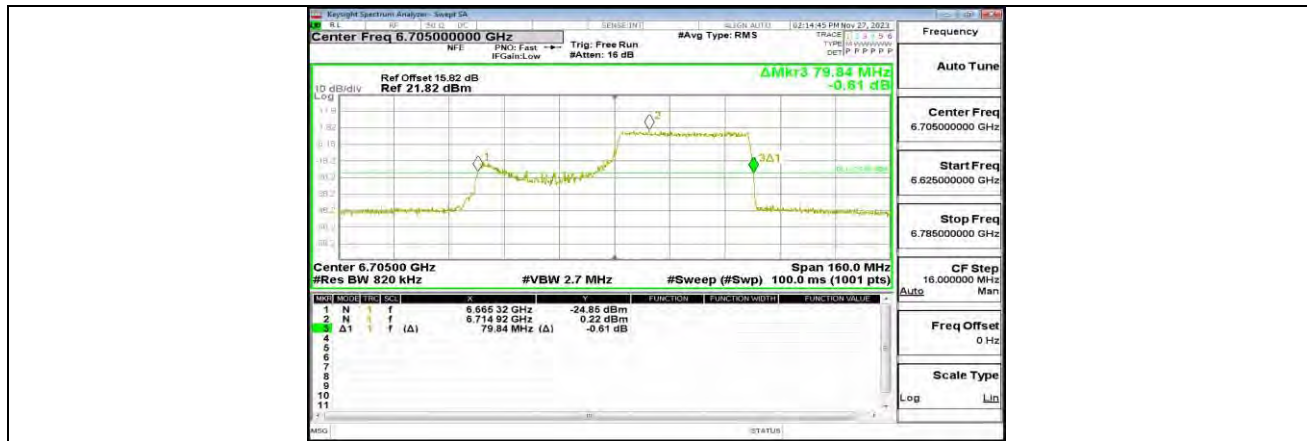
11AX80MIMO_ANT1_6705_484Tone_RU66
