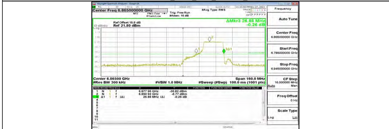
11AX80MIMO_ANT0_6865_242Tone_RU64
