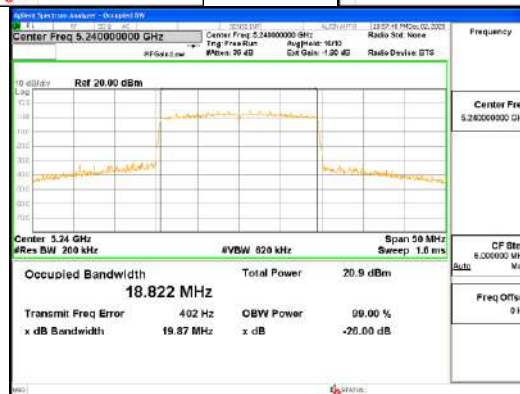
ANT0_802.11ax_HE20_242T_UNII 1
