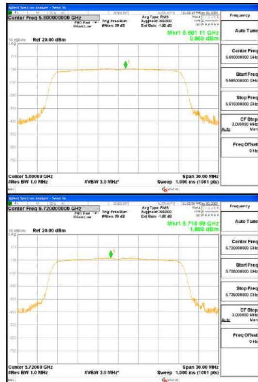
ANT0_802.11ax_HE20_242T_UNII 2C
