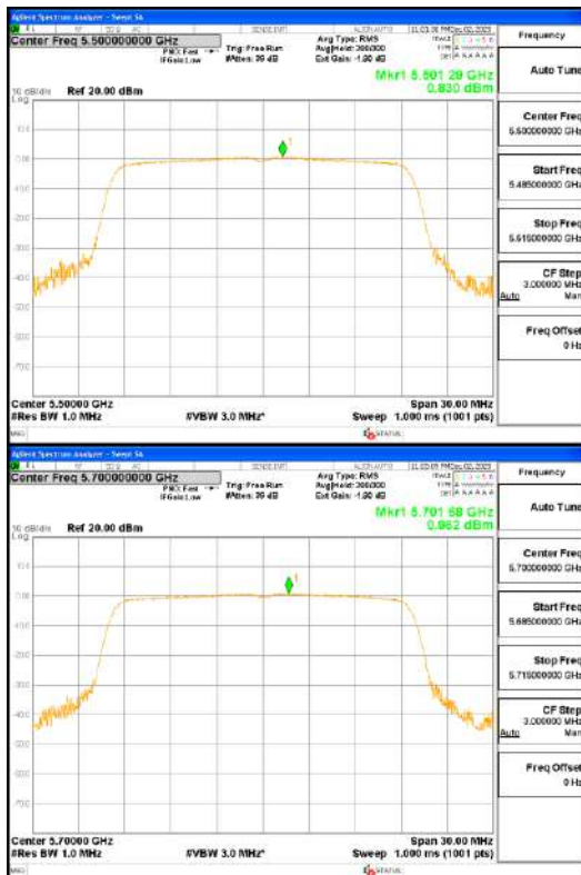
ANT0_802.11ax_HE20_242T_UNII 2C
