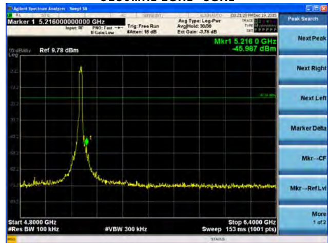
5180MHz 4.8GHz~6.4GHz
