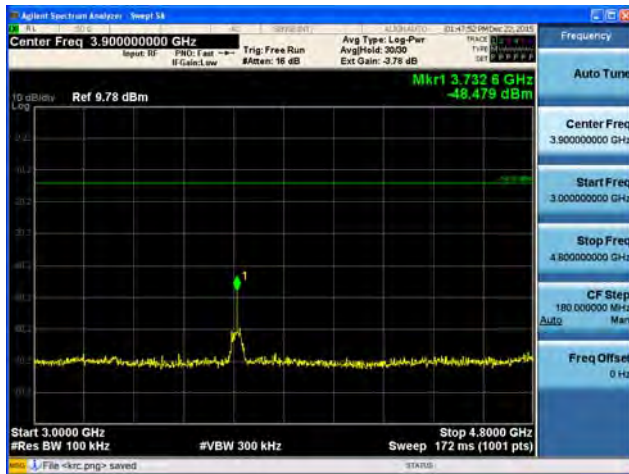
5600MHz 3GHz~4.8GHz
