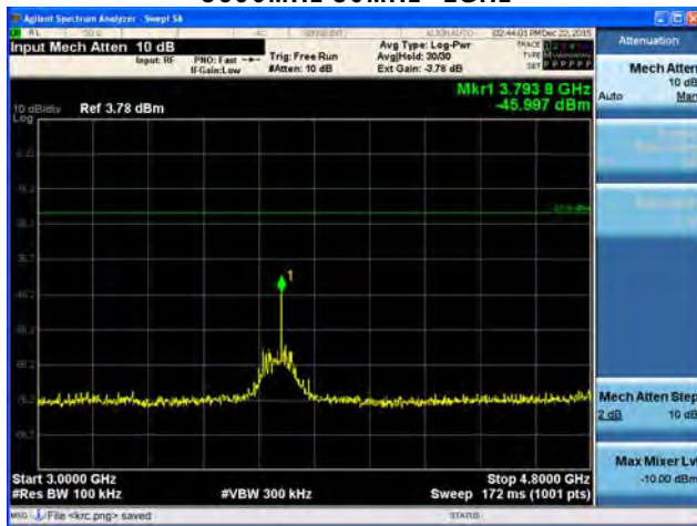
5690MHz 3GHz~4.8GHz
