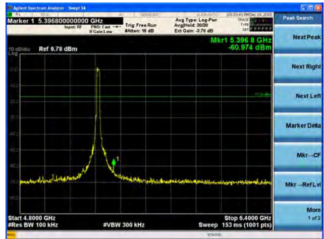
5300MHz 4.8GHz~6.4GHz
