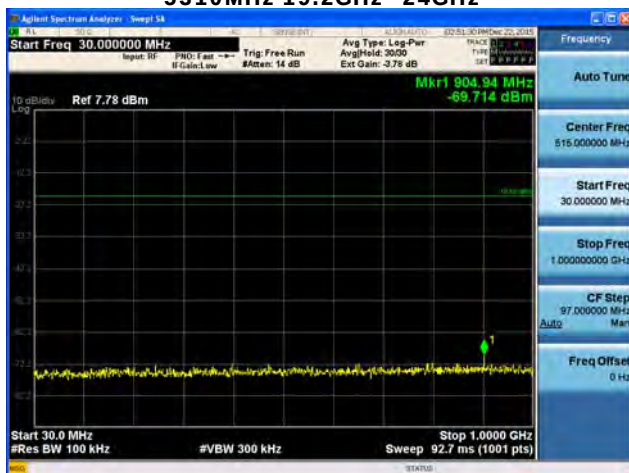
5310MHz 30MHz~1GHz
