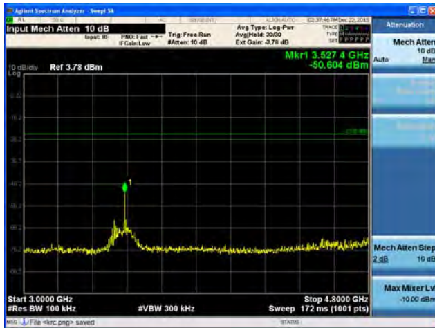
5290MHz 3GHz~4.8GHz
