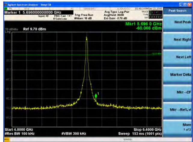
5600MHz 4.8GHz~6.4GHz
