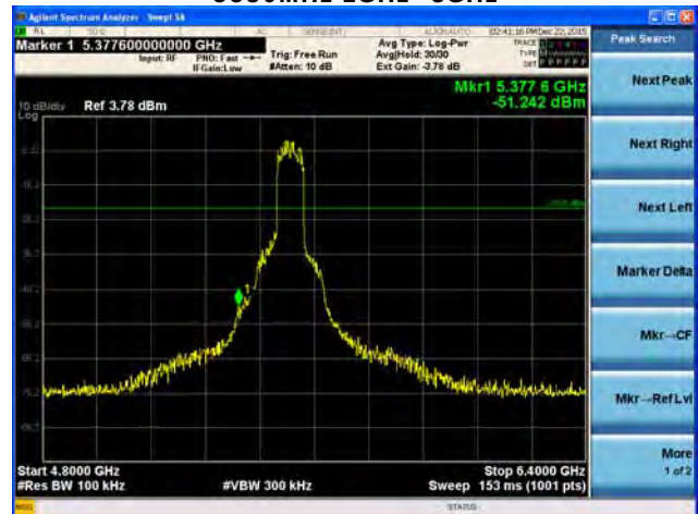
5530MHz 4.8GHz~6.4GHz
