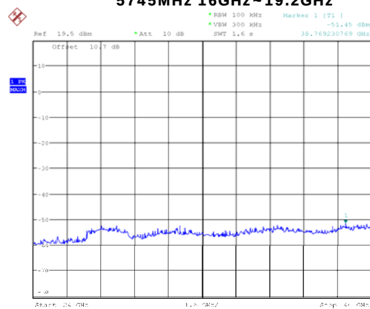
5745MHz 16GHz~19.2GHz
