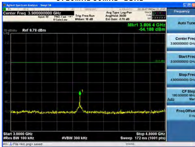
5710MHz 3GHz~4.8GHz
