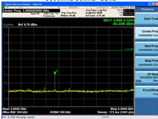
5500MHz 3GHz~4.8GHz
