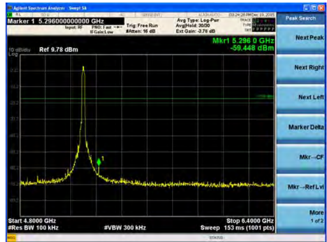
5200MHz 4.8GHz~6.4GHz
