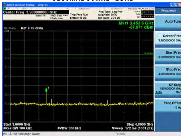
5180MHz 3GHz~4.8GHz
