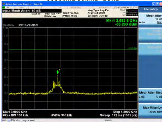
5530MHz 3GHz~4.8GHz
