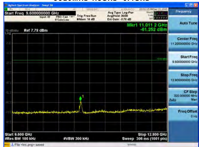
5510MHz 9.6GHz~12.8GHz
