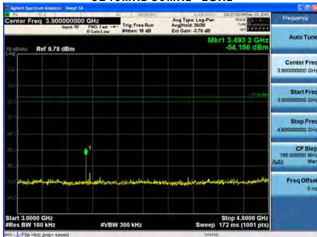
5240MHz 3GHz~4.8GHz
