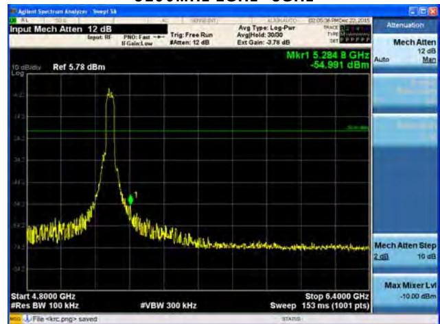
5190MHz 4.8GHz~6.4GHz
