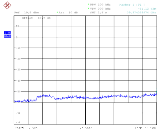
5600MHz 24GHz~40GHz
