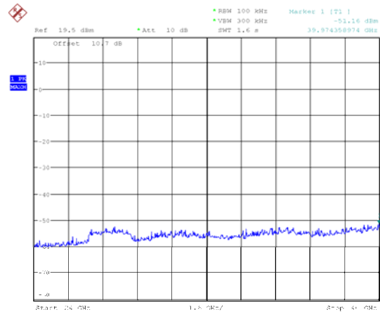
5200MHz 24GHz~40GHz
