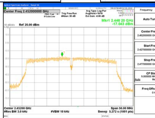
802.11n_HT40_ANT-L
