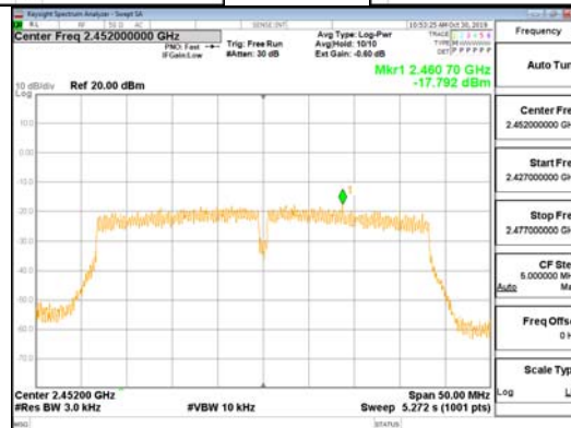
802.11n_HT40_ANT-R
