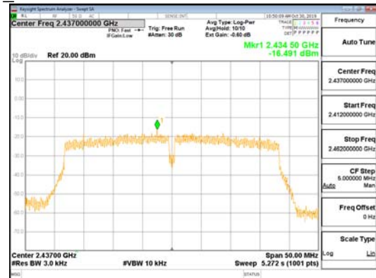
802.11n_HT40_ANT-L
