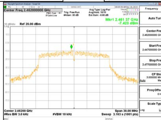
802.11g_ANT-R
