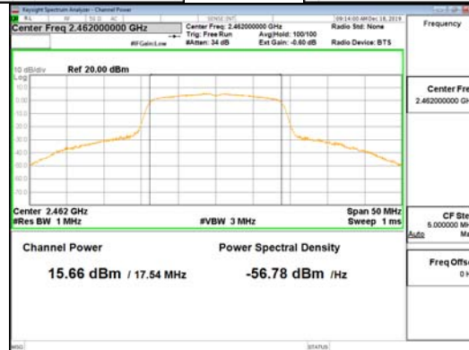
802.11n_HT20_ANT-R
