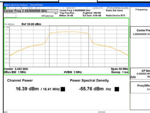
802.11g_ANT-L
