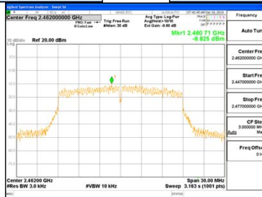
802.11n_HT20_ANT-L
