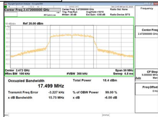
802.11n_HT20_ANT-R
