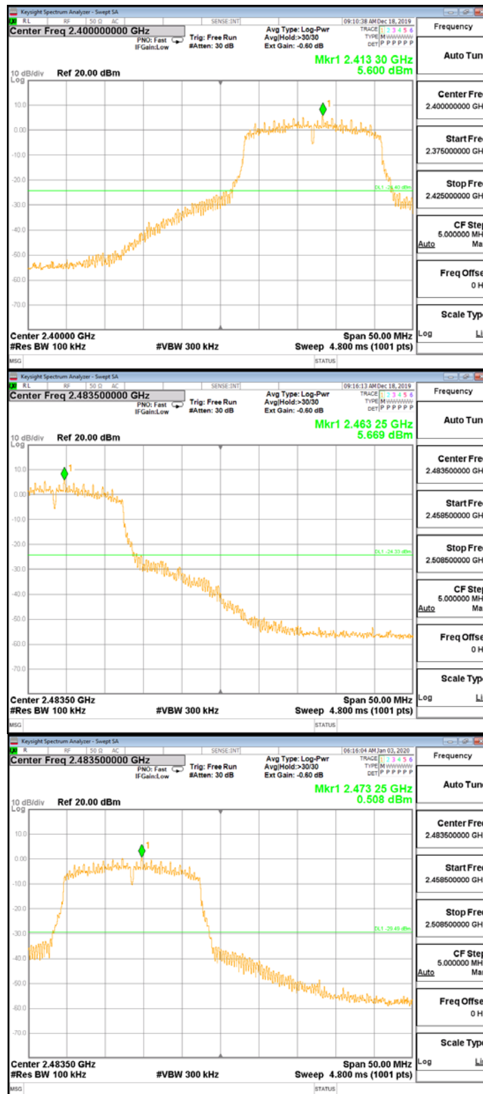
802.11n_HT20_ANT-R
