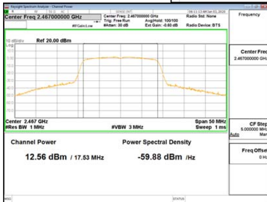
802.11n_HT20_ANT-R
