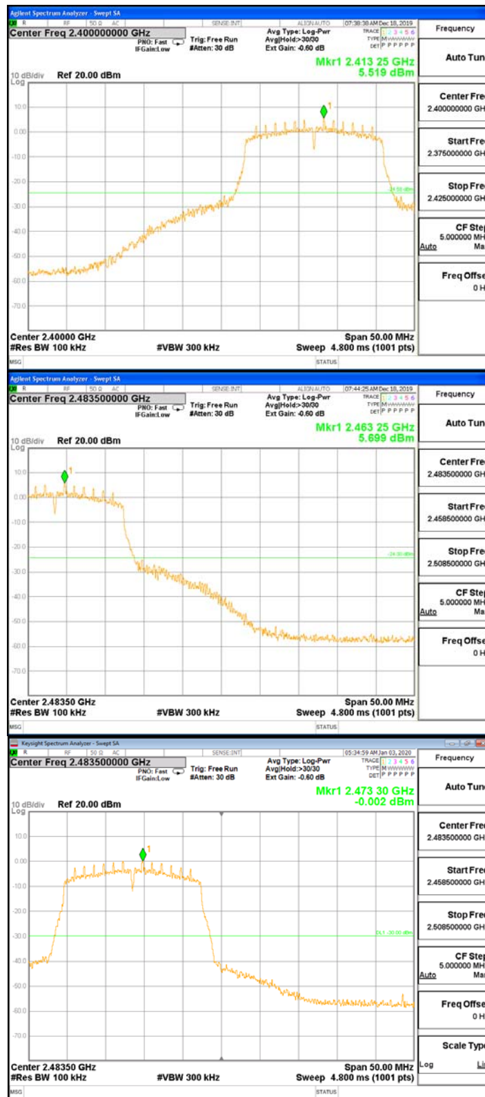
802.11n_HT20_ANT-L
