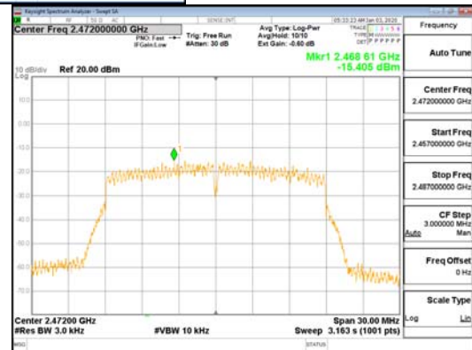
802.11n_HT20_ANT-L
