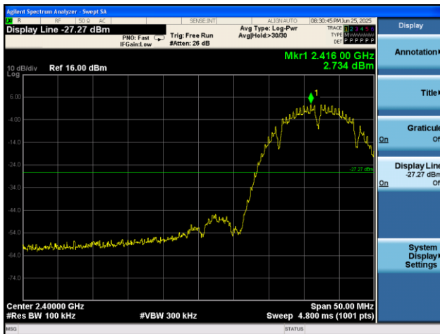
802.11b_2 417 MHz
