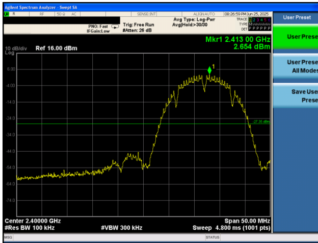
802.11b_2 412 MHz
