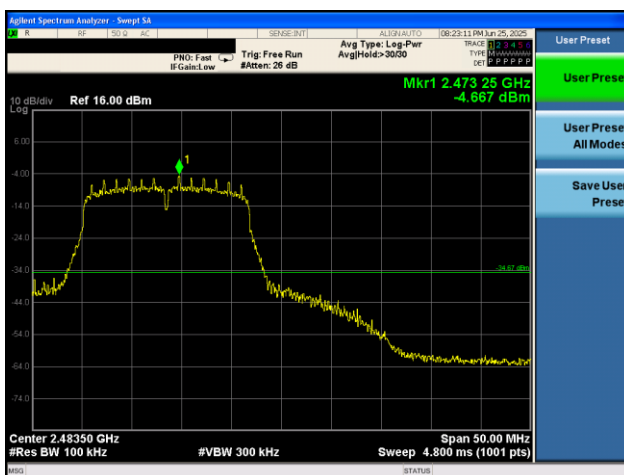
802.11g_2 472 MHz
