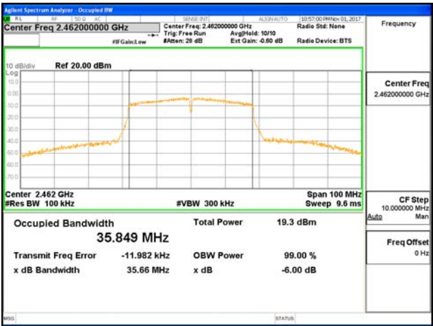
802.11n_HT40_ANT1
