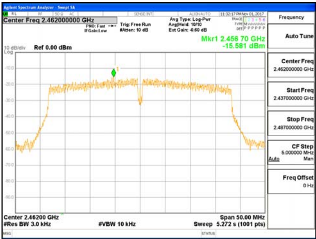
802.11n_HT40_ANT0
