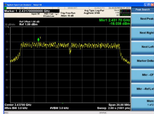
Ant_M2 (2.4GHz) : 802.11b
