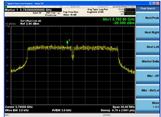
Ant_M1 (5GHz) : 802.11a HT40
