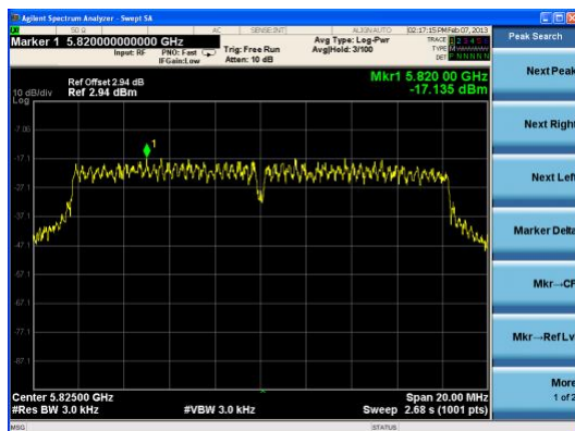
Ant_M1 (5GHz) : 802.11a HT20
