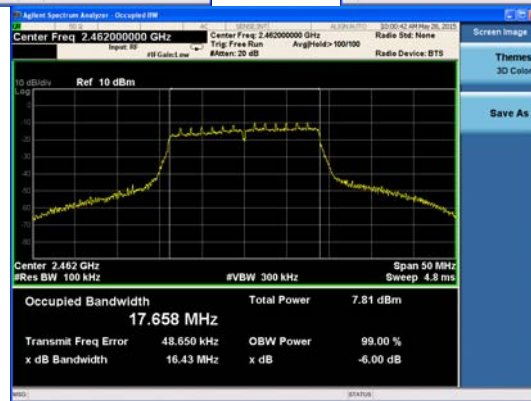
Ant : A2_802.11n
