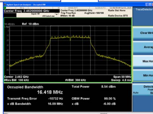
Ant : M1_802.11g
