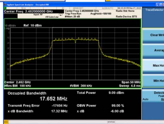
Ant : A1_802.11n
