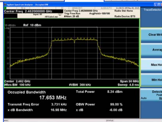
Ant : A3_802.11n
