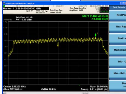
Ant : A2_802.11n
