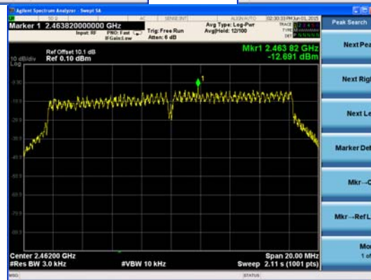
Ant : M2_802.11g
