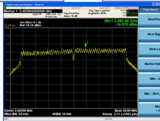
Ant : A2_802.11g
