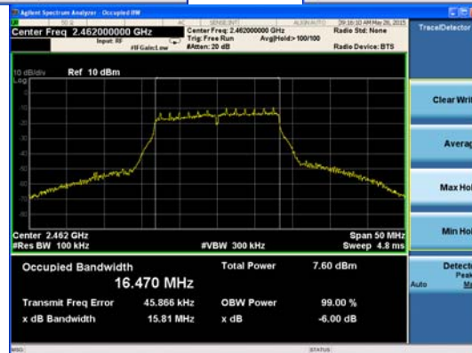
Ant : A2_802.11g
