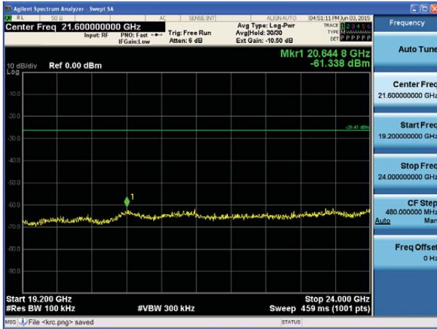
5510MHz 19.2GHz~24GHz
