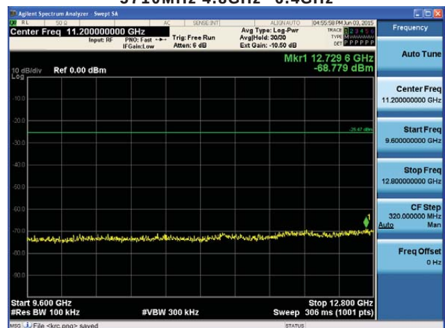
5710MHz 9.6GHz~12.8GHz
