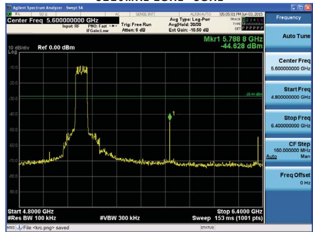
5210MHz 4.8GHz~6.4GHz
