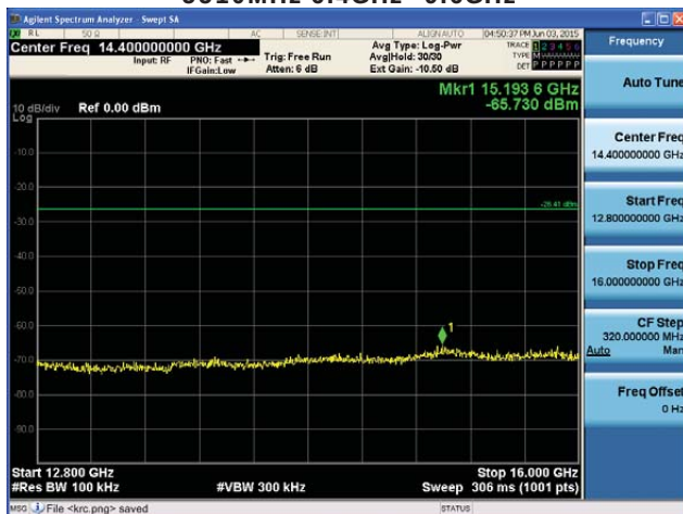
5510MHz 12.8GHz~16GHz
