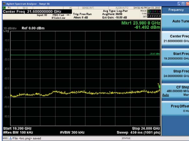
5710MHz 19.2GHz~24GHz
