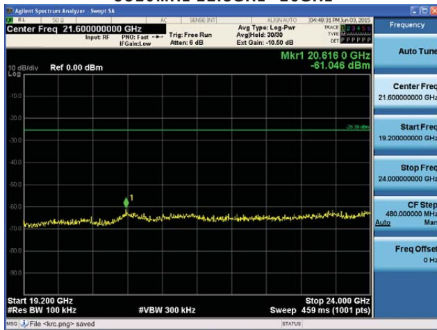
5310MHz 19.2GHz~24GHz
