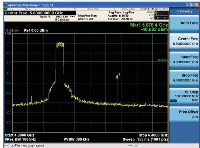
5290MHz 4.8GHz~6.4GHz
