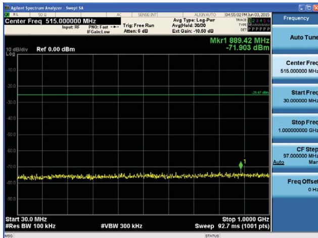
5710MHz 30MHz~1GHz
