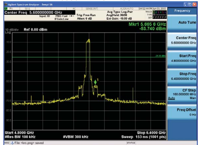
5590MHz 4.8GHz~6.4GHz
