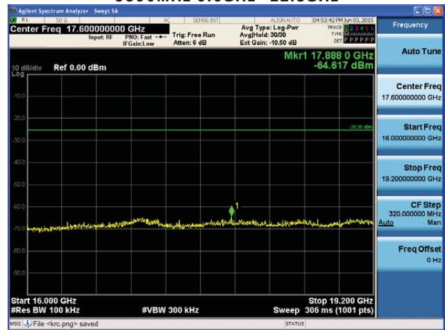
5590MHz 16GHz~19.2GHz
