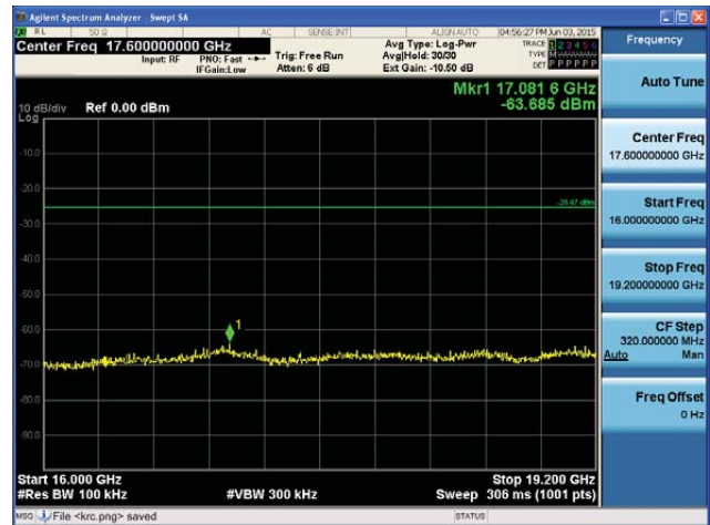
5710MHz 16GHz~19.2GHz
