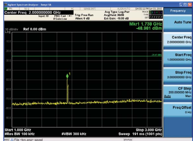
5710MHz 1GHz~3GHz
