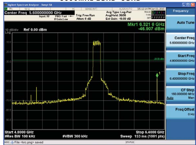
5690MHz 4.8GHz~6.4GHz
