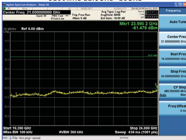
5190MHz 19.2GHz~24GHz
