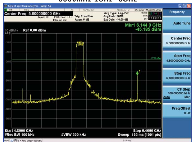
5530MHz 4.8GHz~6.4GHz
