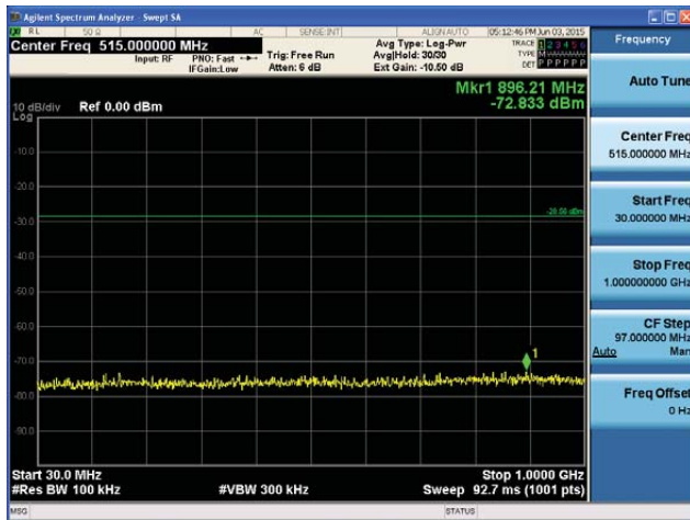
5690MHz 30MHz~1GHz
