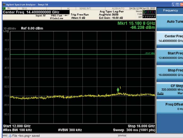
5710MHz 12.8GHz~16GHz
