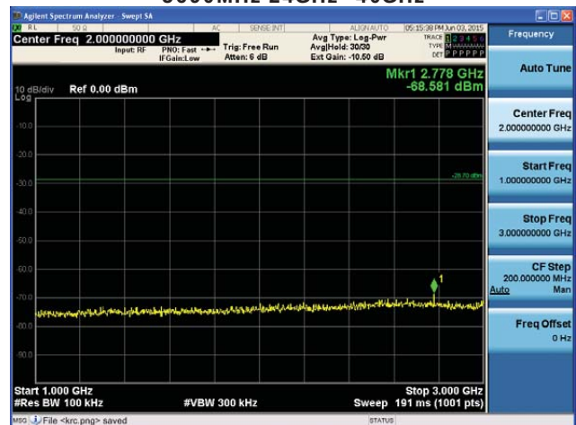
5775MHz 1GHz~3GHz
