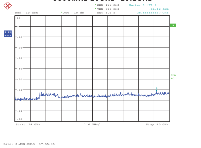
5500MHz 24GHz~40GHz
