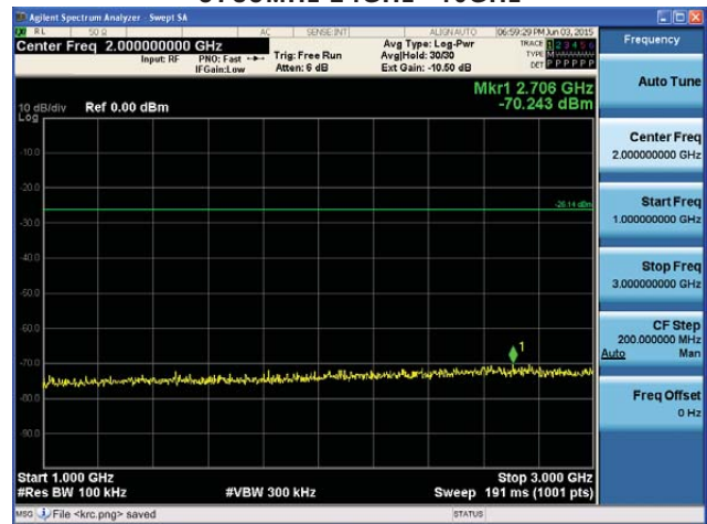
5825MHz 1GHz~3GHz
