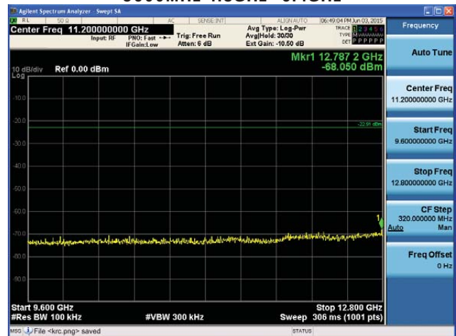
5600MHz 9.6GHz~12.8GHz
