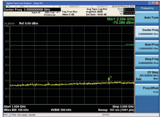
5720MHz 1GHz~3GHz
