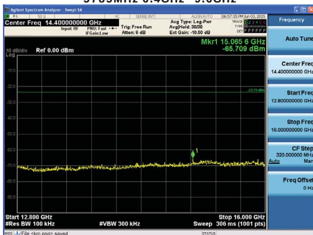
5785MHz 12.8GHz~16GHz
