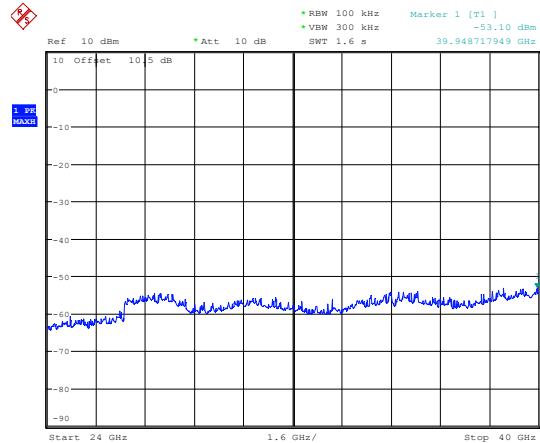
5690MHz 24GHz~40GHz
