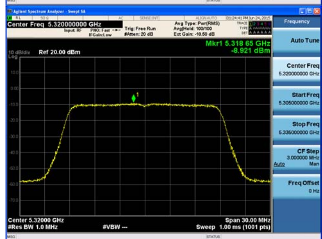
Ant : A2_802.11ac_VHT20 (1)
