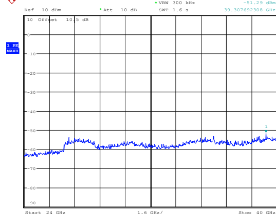
5300MHz 24GHz~40GHz
