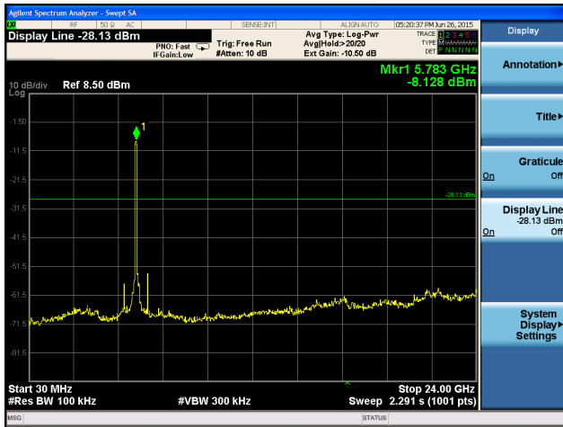
5775MHz 30MHz~24GHz
