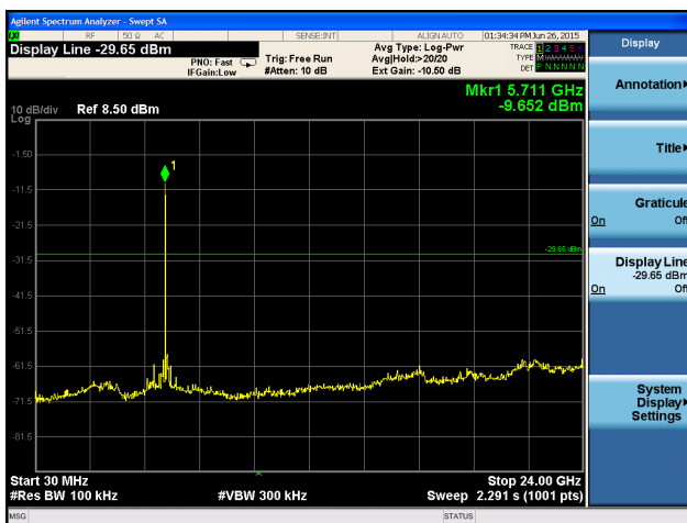
5720MHz 30MHz~24GHz
