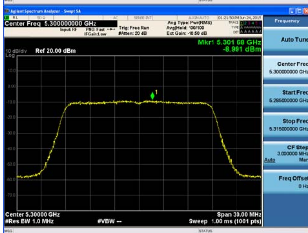
Ant : A2_802.11ac_VHT20 (1)
