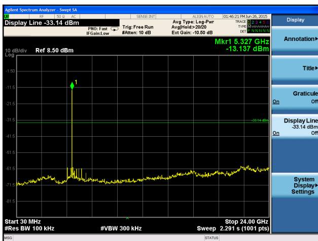
5320MHz 30MHz~24GHz
