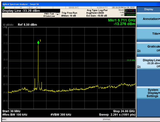
5690MHz 30MHz~24GHz
