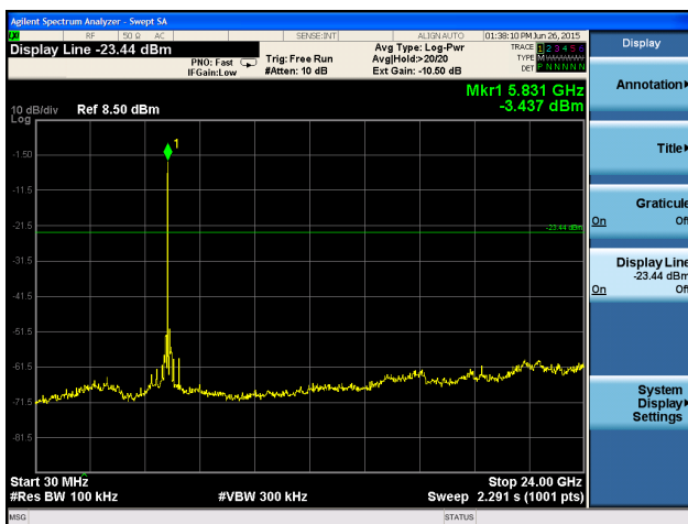
5825MHz 30MHz~24GHz
