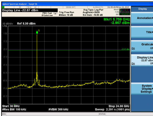
5745MHz 30MHz~24GHz
