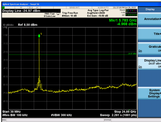
5785MHz 30MHz~24GHz
