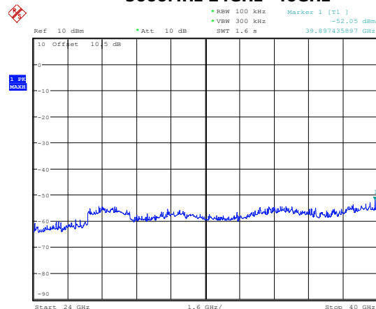
5600MHz 24GHz~40GHz
