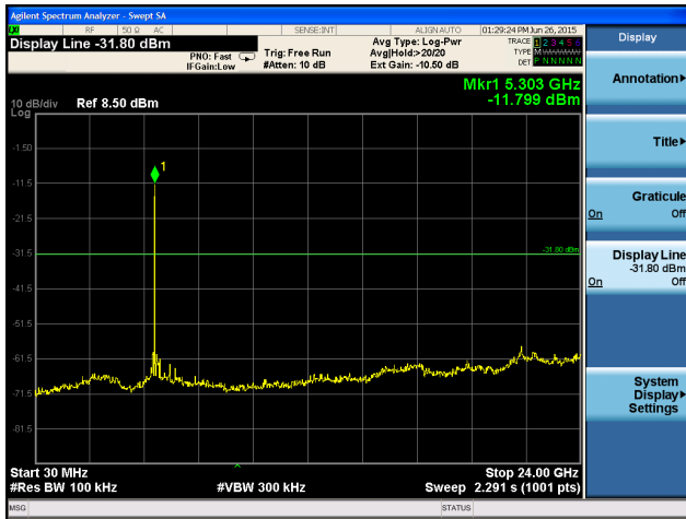
5300MHz 30MHz~24GHz
