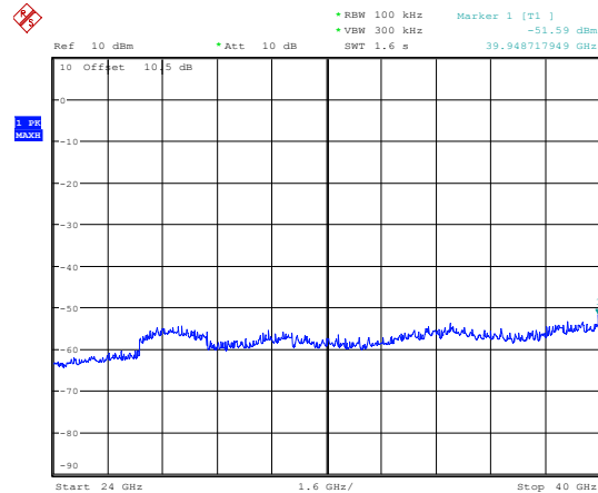
5500MHz 24GHz~40GHz
