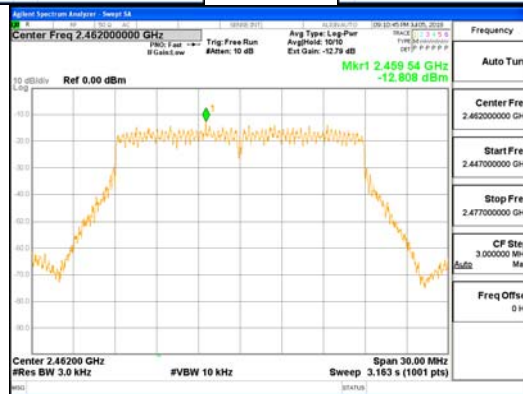
802.11n_HT20_ANT0
