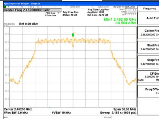
802.11n_HT20_ANT3
