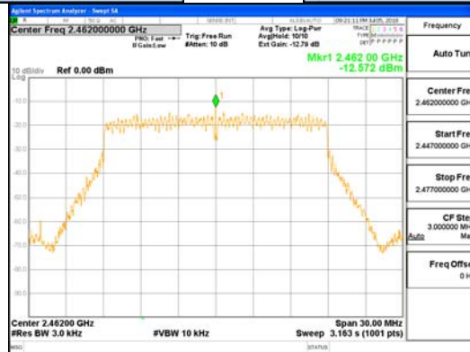
802.11n_HT20_ANT1
