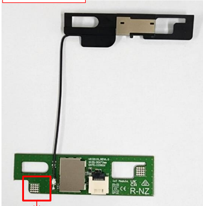
ANT & PCB
