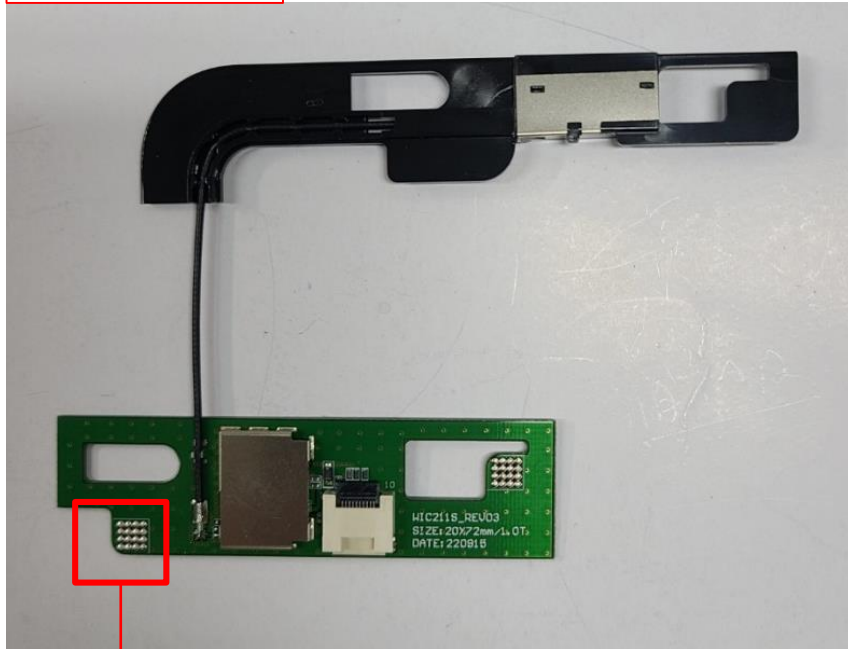
ANT & PCB
