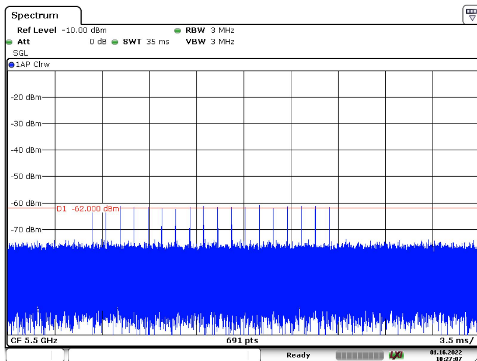
Radar Type 1A – 5500MHz
