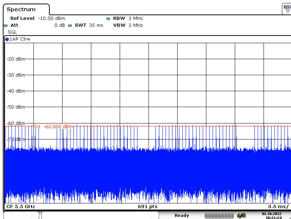
Radar Type 3 – 5500MHz
