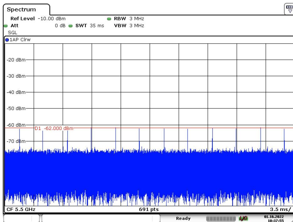
Radar Type 5 – 5500MHz
