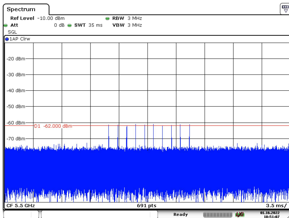
Radar Type 1B – 5500MHz
