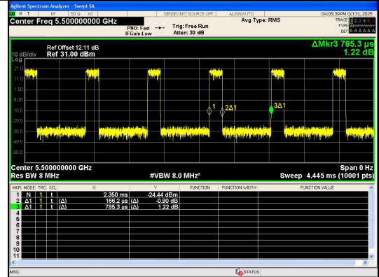
IEEE 802.11n 20MHz Channel 100
