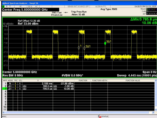
IEEE 802.11n 20MHz Channel 120
