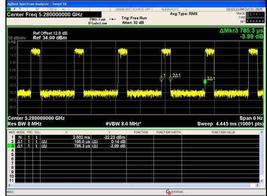
IEEE 802.11n 20MHz Channel 56
