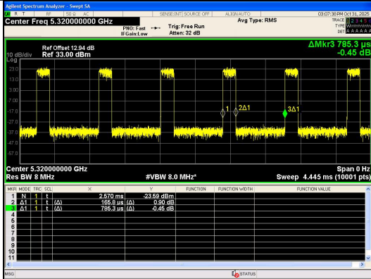
IEEE 802.11n 20MHz Channel 64
