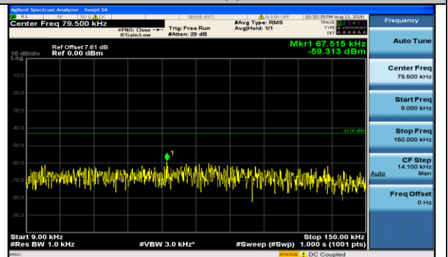
Band66-20MHz-QPSK-132572-1RB#0-0.009~0.15-PASS
