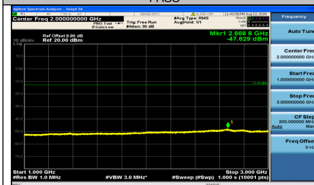
Band71-20MHz-QPSK-133372-100RB#0-1000~3000-PASS
