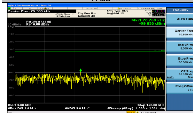
Band71-20MHz-QPSK-133372-100RB#0-0.009~0.15-PASS
