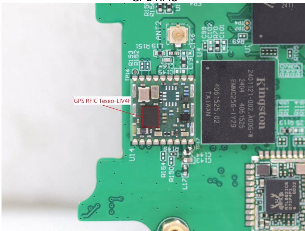
GPS RFIC
