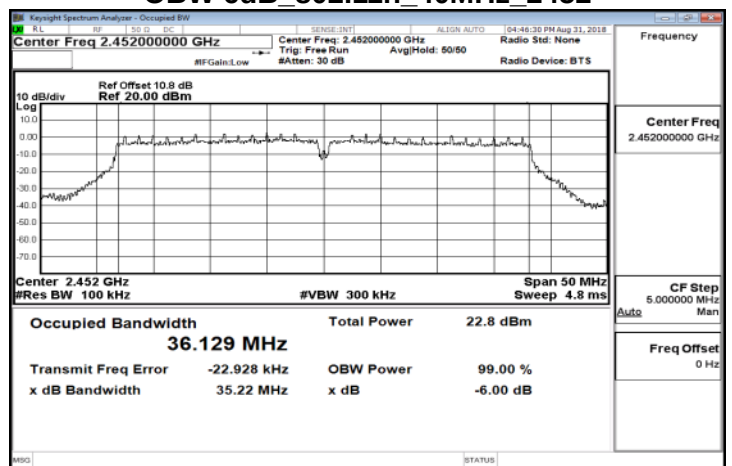
OBW 6dB 802.11n 40MHz 2452
