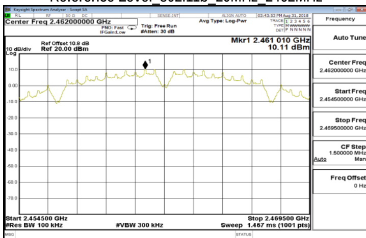
Reference Level 802.11b 20MHz 2462MHz
