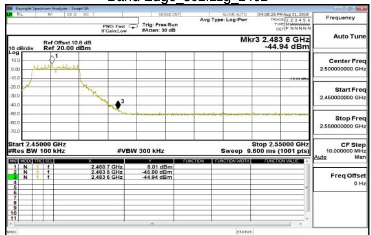
Band Edge 802.11g 2462
