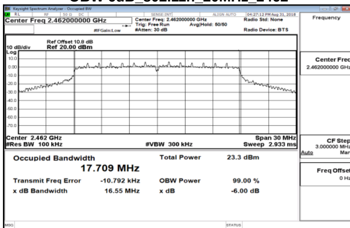
OBW 6dB 802.11n 20MHz 2462
