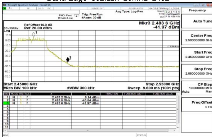
Band Edge 802.11n 20MHz 2462
