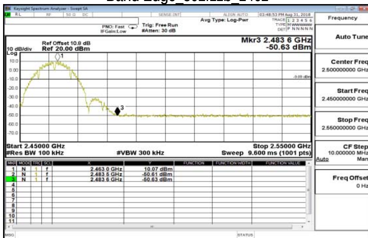
Band Edge 802.11b 2462
