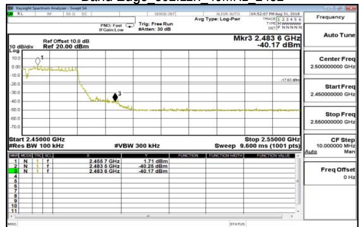
Band Edge 802.11n 40MHz 2452
