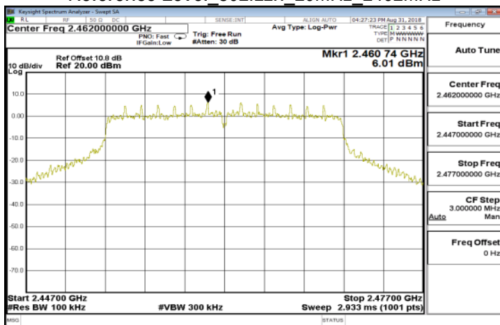
Reference Level 802.11n 20MHz 2462MHz
